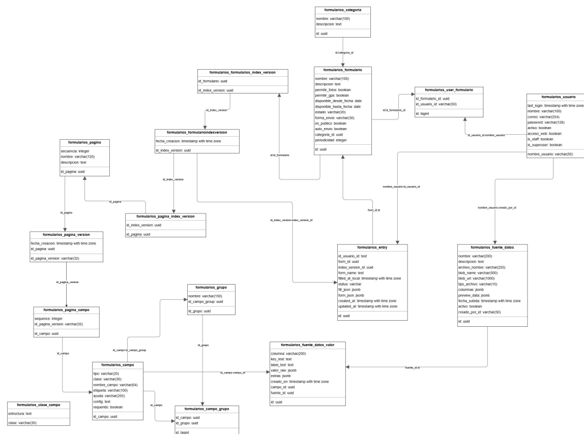
Figura 1: Modelo entidad–relación de la base de datos utilizada para formularios adaptables.
