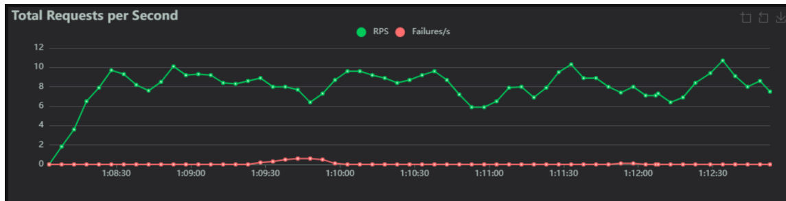
Figura 7: Requests por segundo (RPS) y fallos por segundo (Failures/s) con 80 usuarios.
