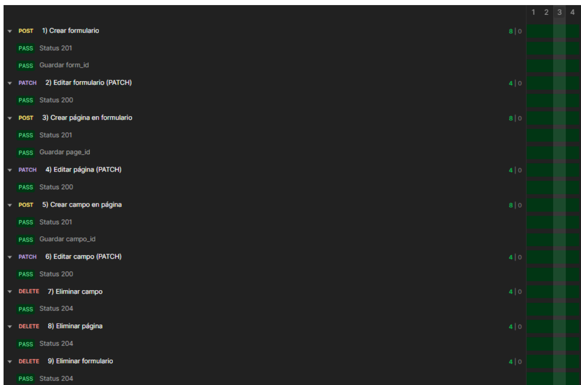
Figura 3: Ejecución de la colección Postman ( CRUD Flow )
