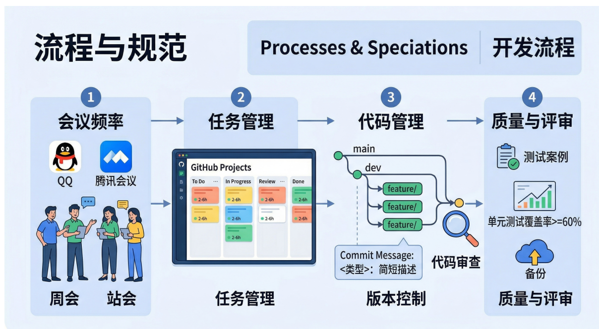
图 2: 开发流程图
