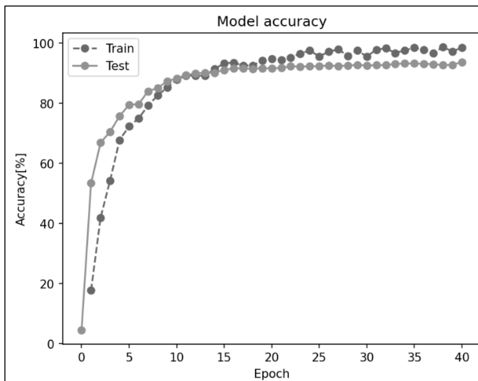
図 128 学習率 0.001、エポック 40、拡張した学習データを用いた CNN モデル 5 のエポックと精度のグラフ
