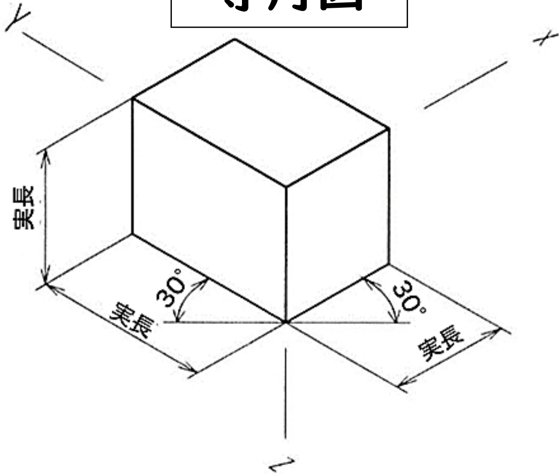
等角図
