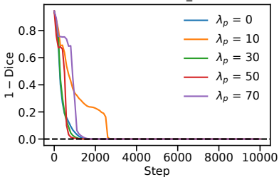
Dice Loss (bud_04)
