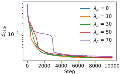
Data Loss (multi)
