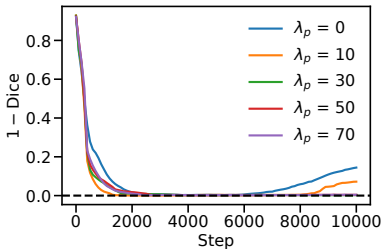
Dice Loss (biconcave)
