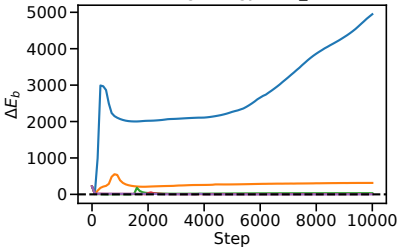
Bending Energy (bud_04)
