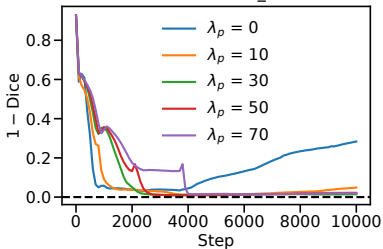
Dice Loss (bud_04)
