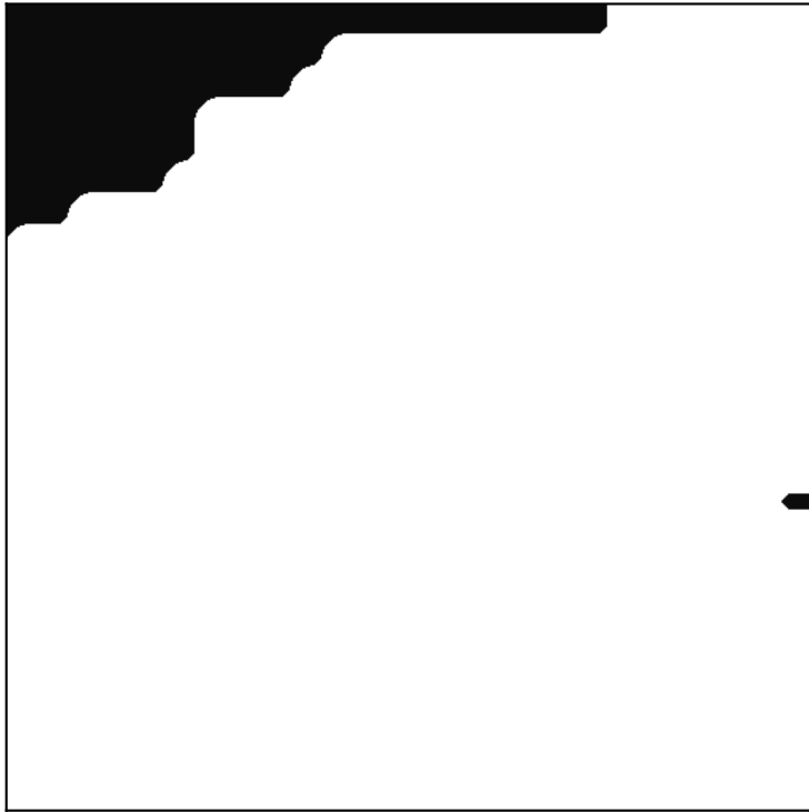
MAJA
