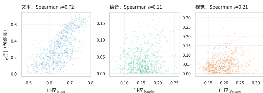
图 5.12 门控——贡献一致性散点（附件 2 验证集，728 条，分模态）
