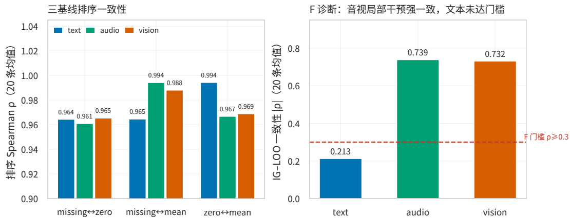
图 5.10 IG 验证与 F 项诊断 (三基线排序一致性)
