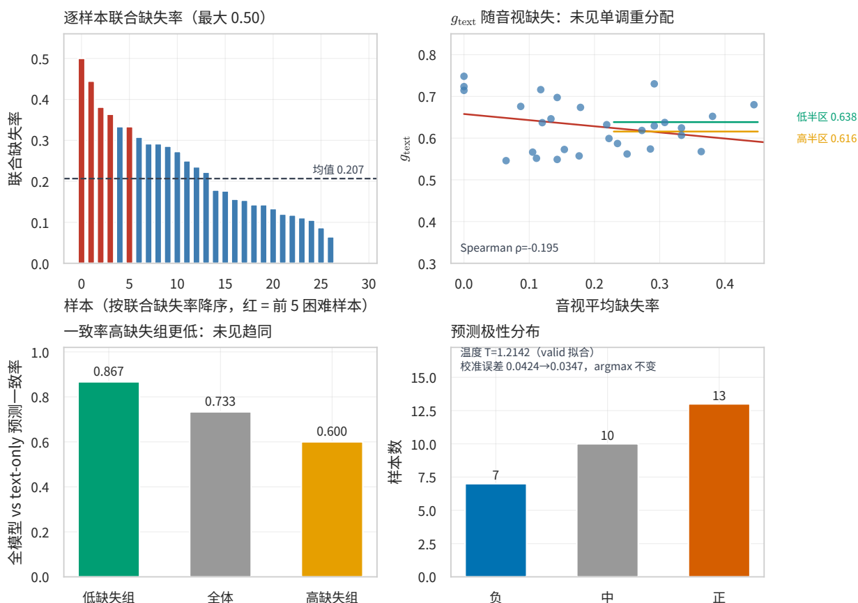
图 4.8 附件 3 行为分析（MRFN+ 集成，30 条，无标签）
