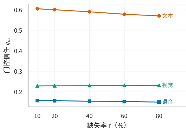
图 4.7 门控信任随缺失率的响应（验证集，三种子均值）
