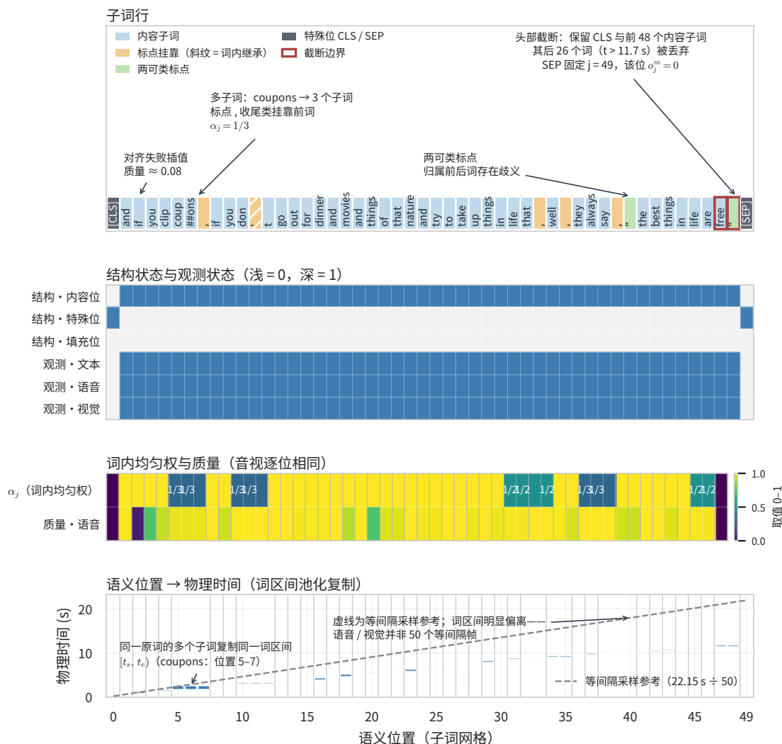
图 3.3 50 位语义网格与状态标注（截断样本示例）
