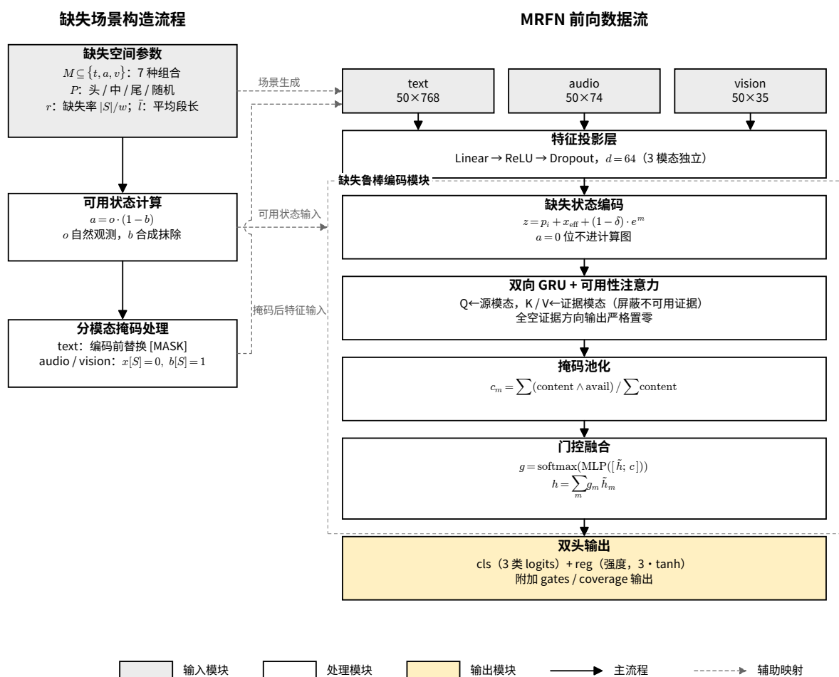
图 4.5 MRFN 缺失场景构造与数据流（左：三级构造；右：四阶段）
