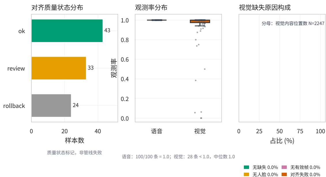
图 3.4 问题一验收三联图：对齐质量、观测率与缺失原因
