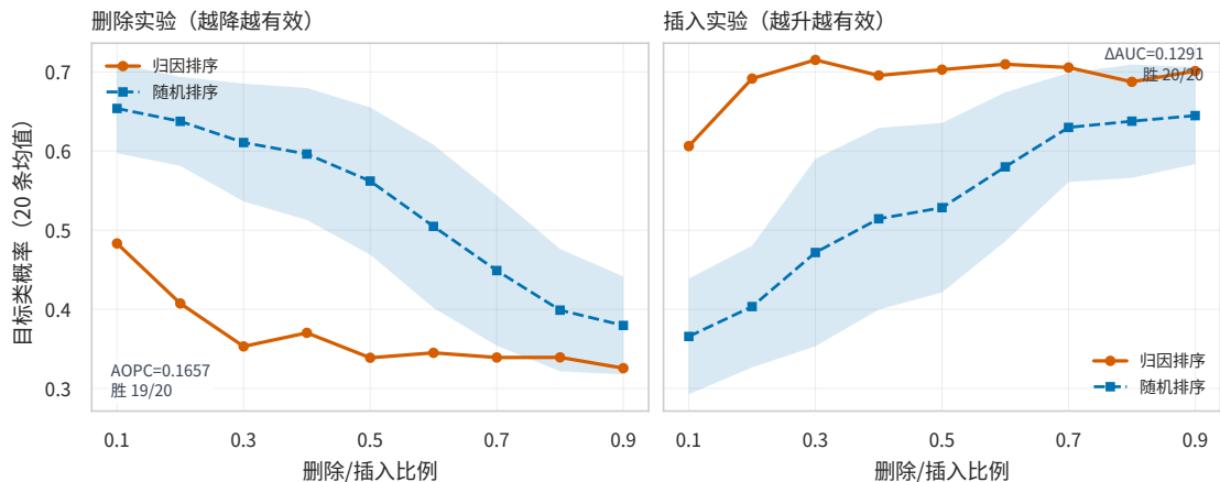
图 5.11 删除/插入保真度曲线（归因序与随机序对照）
