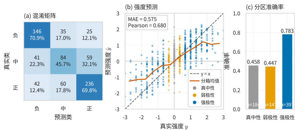
图 7.1 MRFN+ 双输出性能与误差结构
