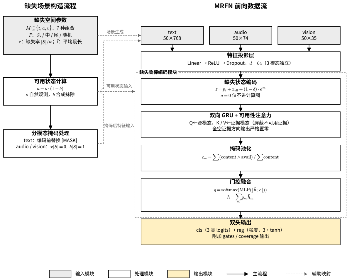
图 5.2 MRFN 缺失场景构造与数据流
