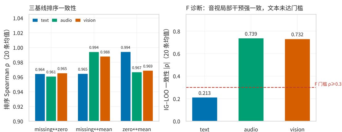
图 6.4 IG 验证与 F 项诊断
