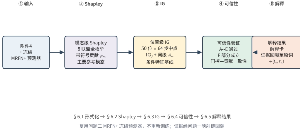
图 6.1 问题三求解流程
