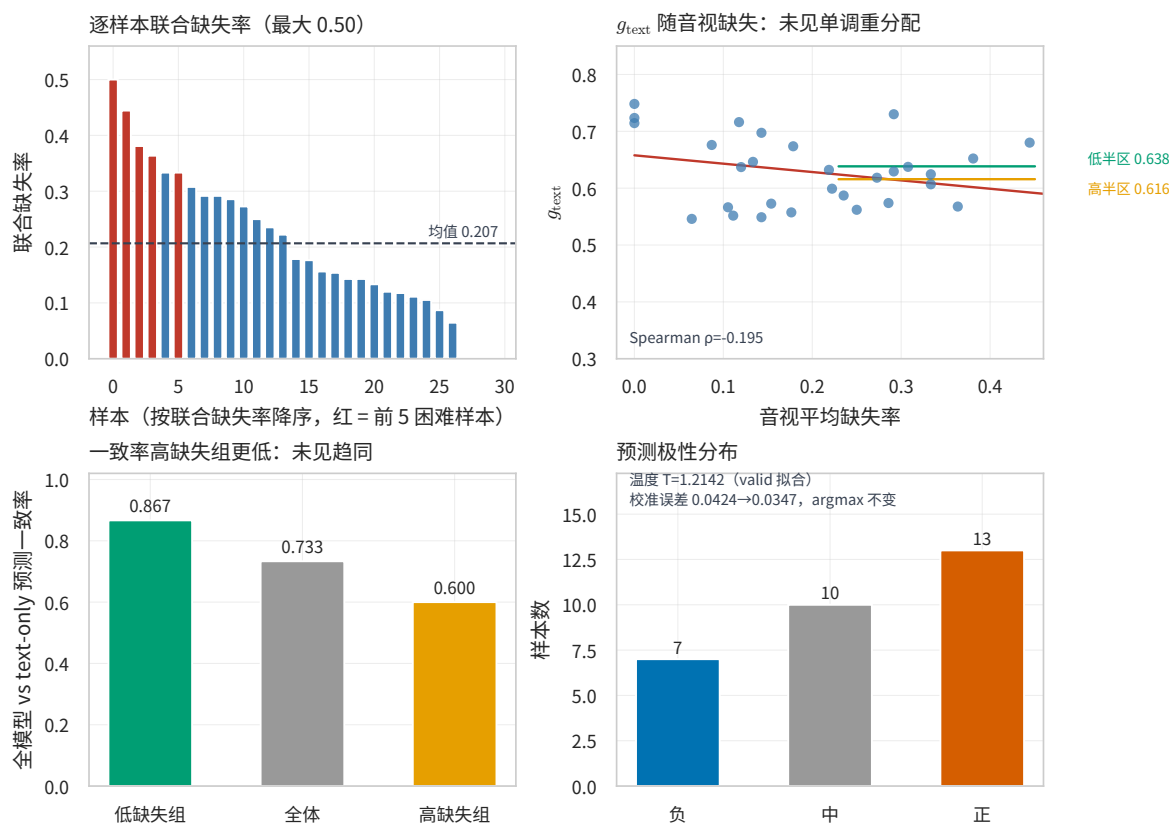
图 5.7 附件 3 行为分析
