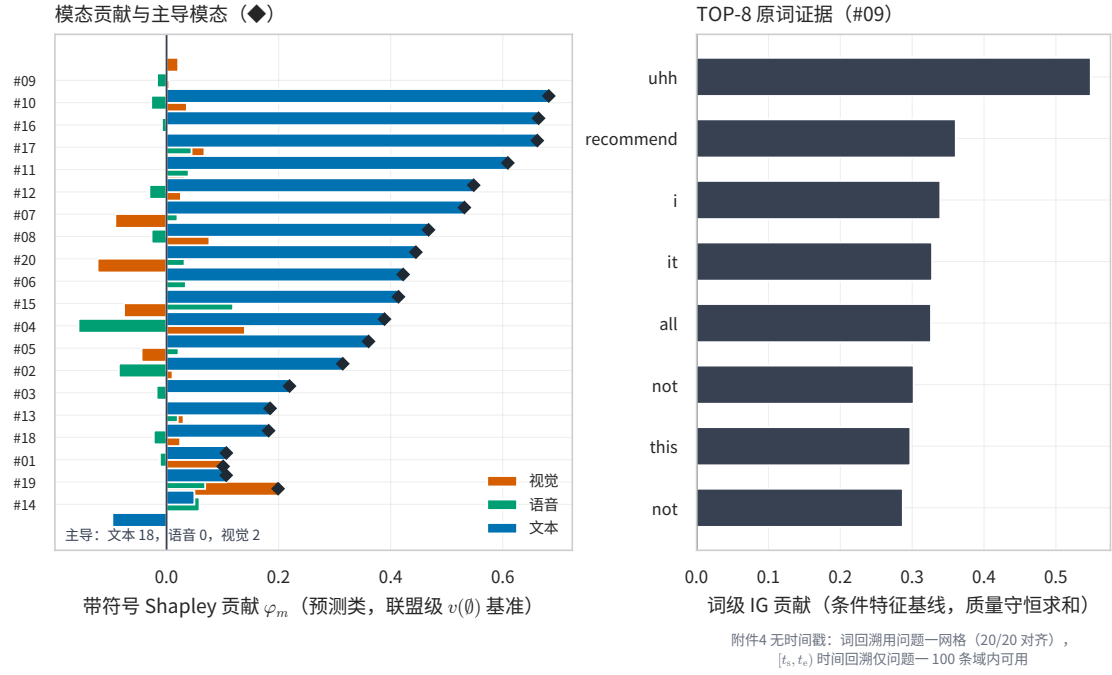
图 6.2 模态贡献与词级证据回溯
