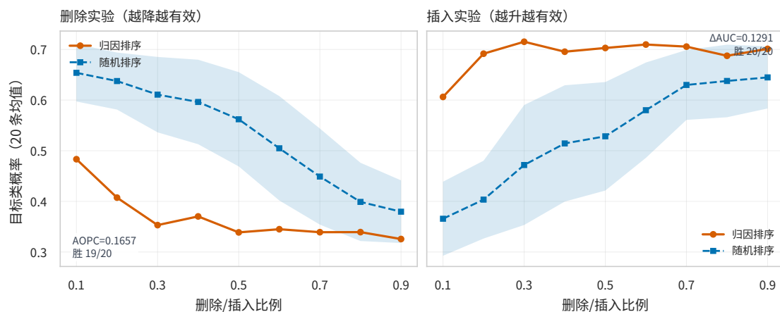
图 6.6 删除/插入保真度曲线
