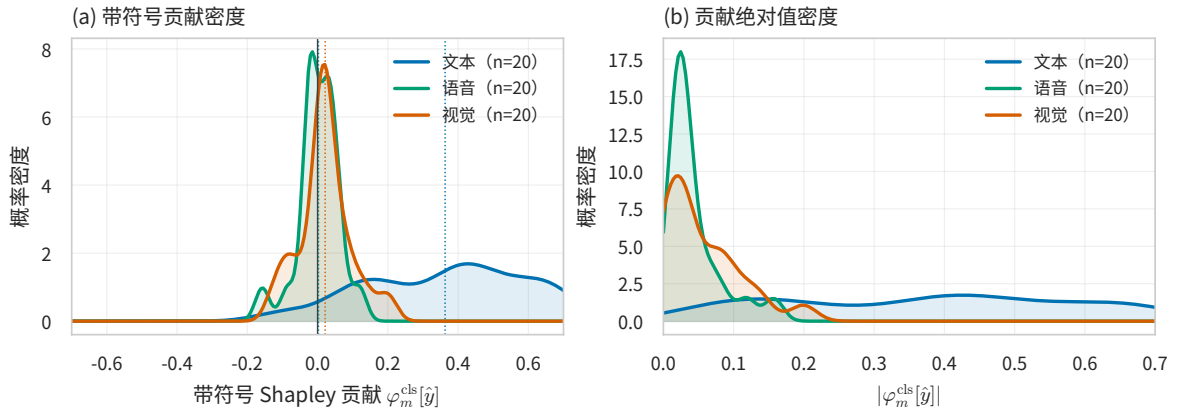
图 6.3 三模态 Shapley 贡献密度
