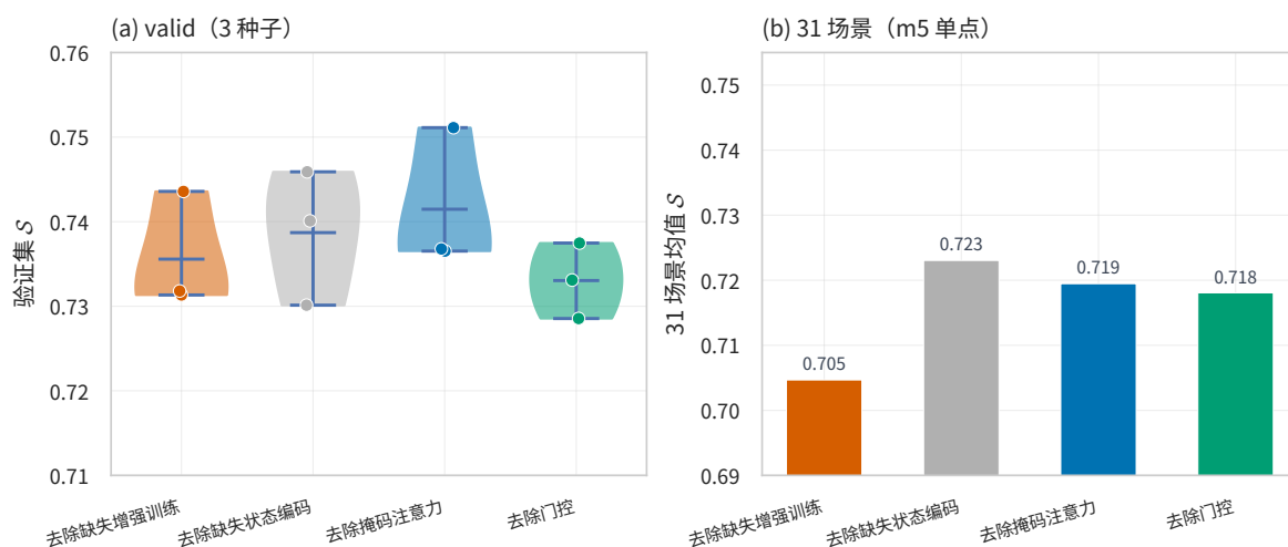
图 7.2 四项消融变体的性能分布
