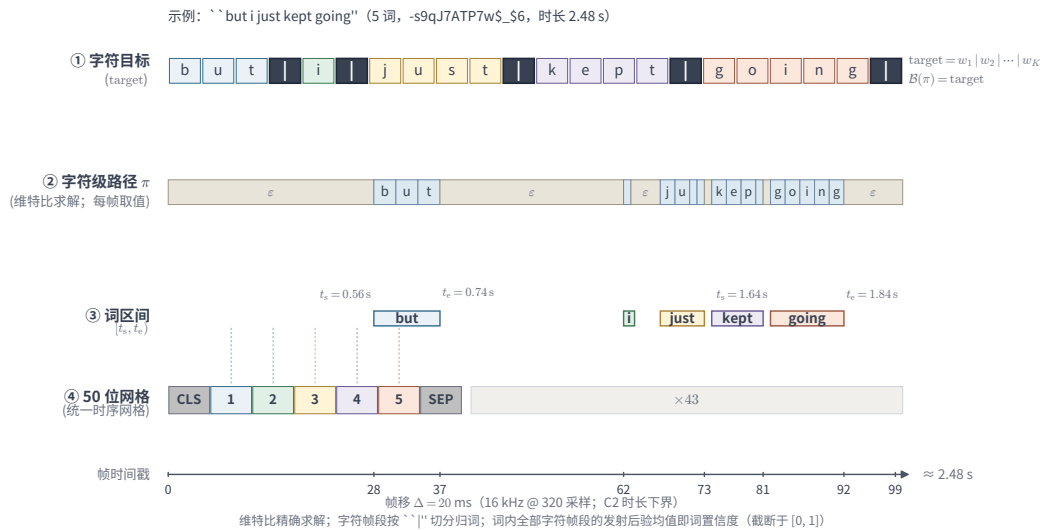
图 4.6 CTC 逐步对齐示例
