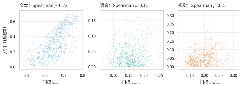
图 6.7 门控—贡献一致性散点
