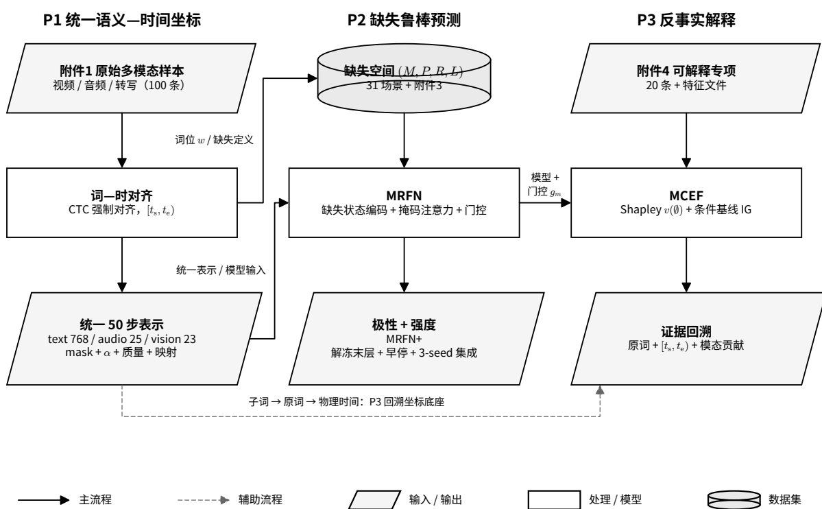
图 2.2 全文总体技术路线
