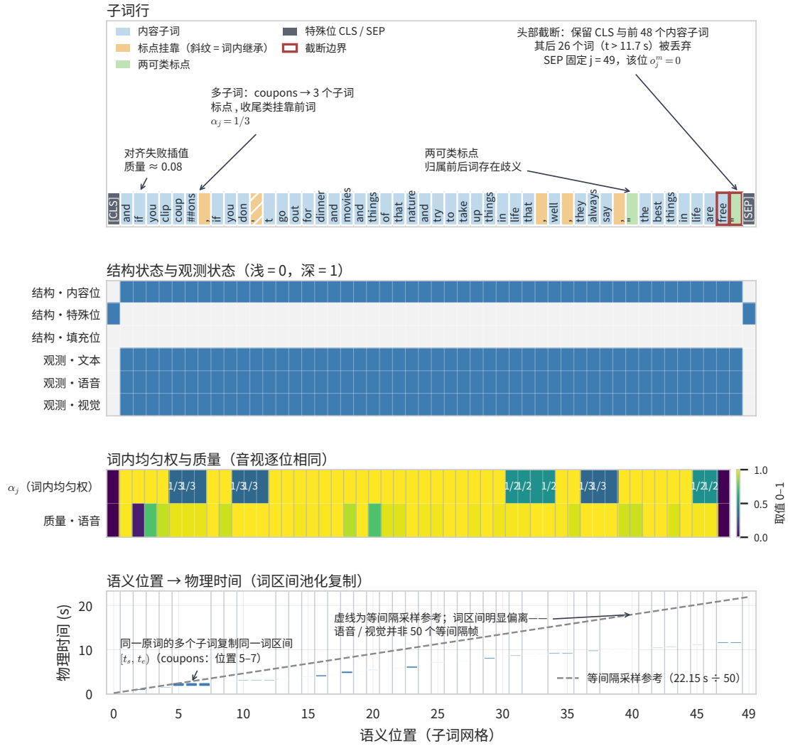
图 4.5 50 位语义网格与状态标注
