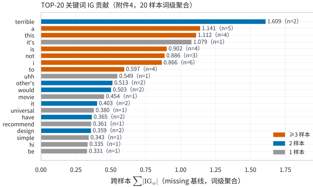
图 6.5 TOP-20 关键词 IG 贡献
