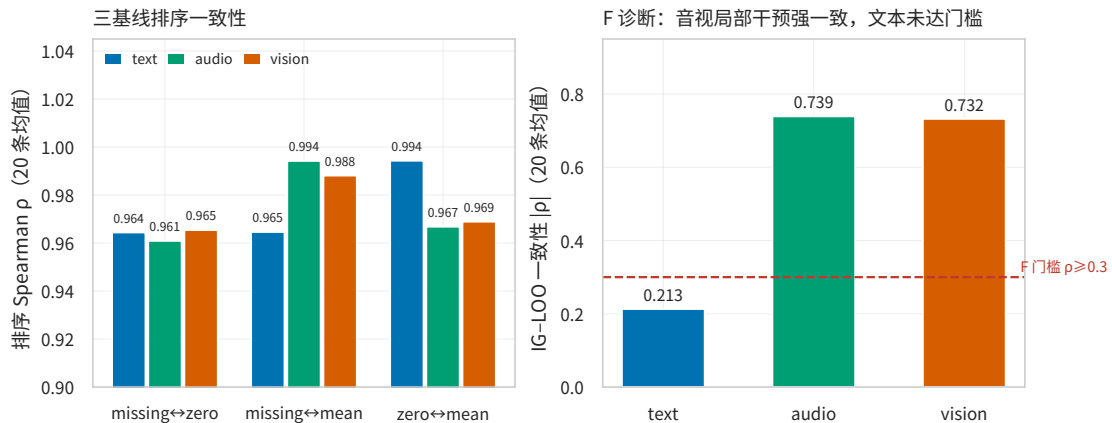
图 6.12 IG 验证与 F 项诊断 (三基线排序一致性)
