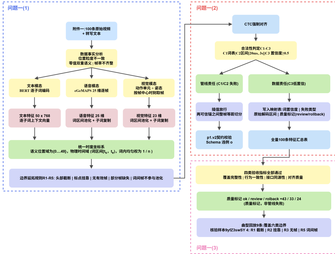
图 3.2 问题一求解流程：原始素材 → 子词化与特征提取 → CTC 强制对齐 → 统一时序坐标 → 四类机器指标验收
