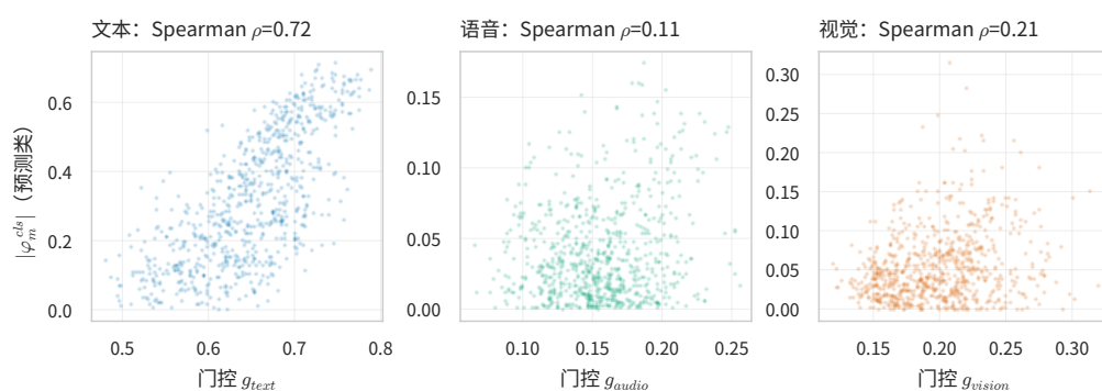
图 6.14 门控——贡献一致性散点（附件 2 验证集，728 条，分模态）
