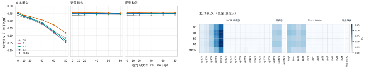
图 4.8 缺失场景实验结果: (a) 退化曲线; (b) D_S 热力图
