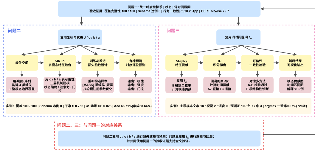
图 4.6 问题二求解流程：缺失空间定义 → MRFN 三层机制 → 训练与阶梯 → 31 场景鲁棒性评测 → 改进采纳与附件 3 预测
