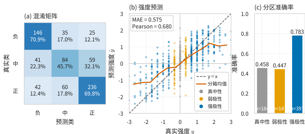
图 6.16 MRFN+ 双输出性能与误差结构（附件 2 验证集，728 条）
