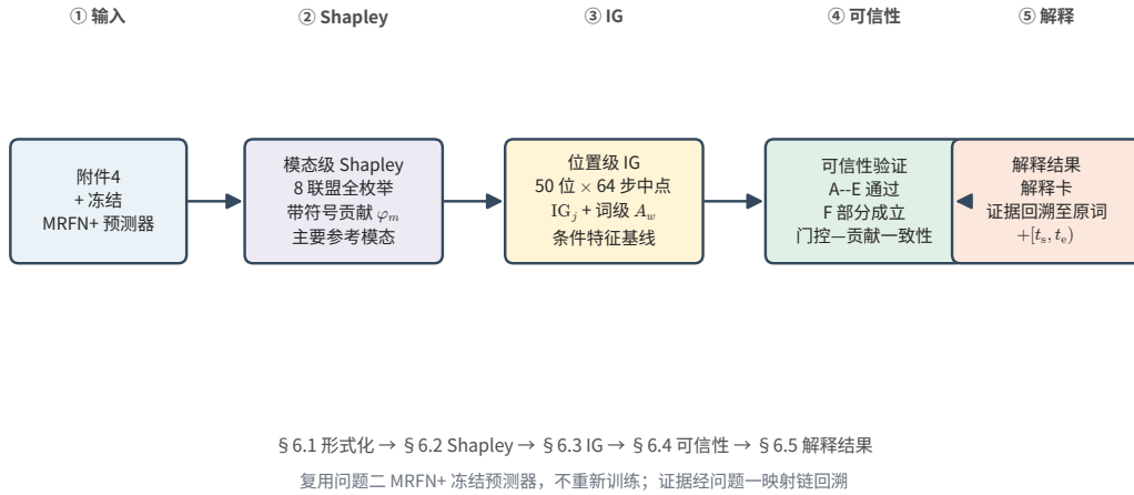
图 5.11 问题三求解流程：解释任务形式化 → 模态级 Shapley → 位置级 IG → 六项保真度检验 → 附件 4 证据回溯
