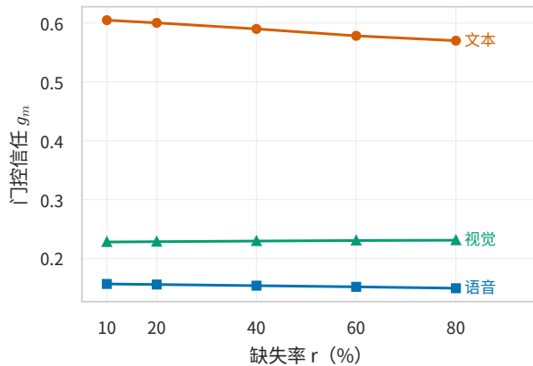
图 4.9 门控信任随缺失率的响应（验证集，三种子均值）
