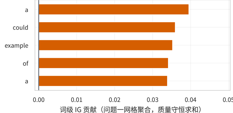
词级 IG 贡献（问题—网格聚合，质量守恒求和）
