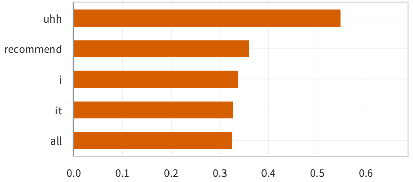
TOP-5 原词证据（IG，条件特征基线）
