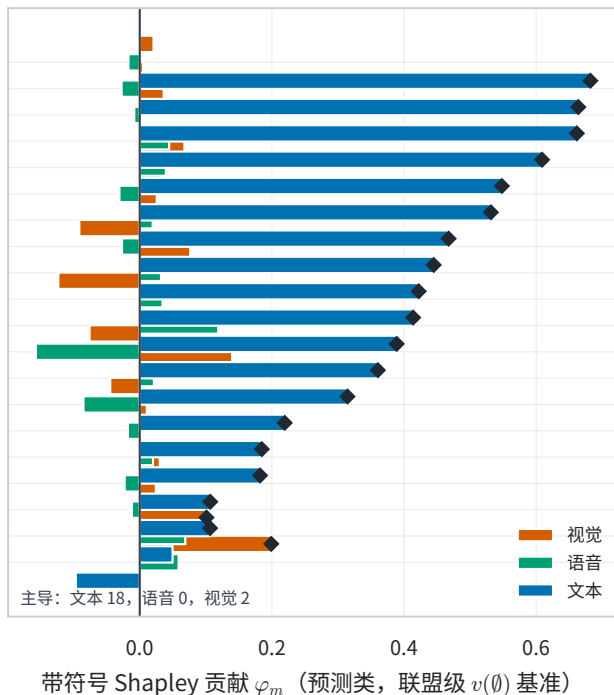
模态贡献与主导模态 (◆)
