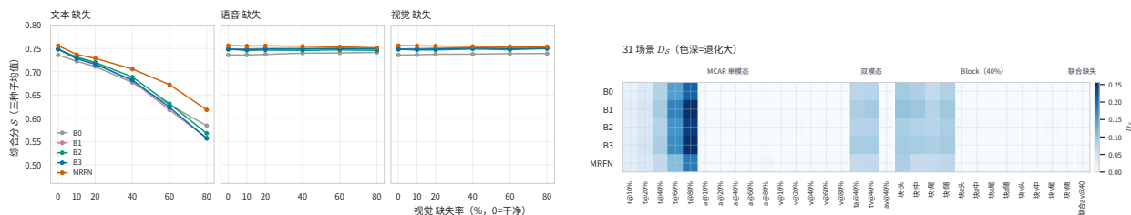
图 5.6 缺失场景实验结果: (a) 退化曲线; (b) D_S 热力图
