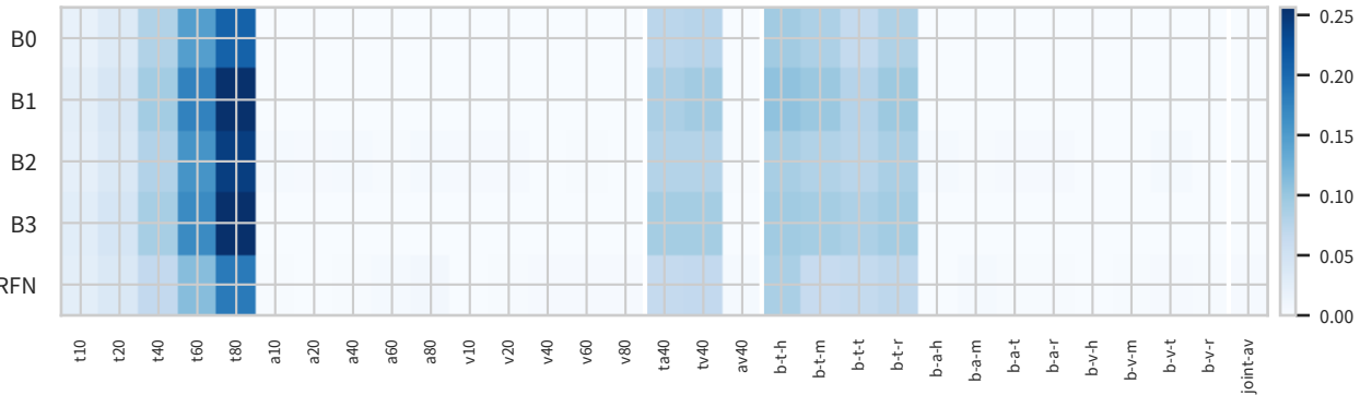
31 缺失场景下的性能退化 D_S (3-seed 均值; 颜色越深退化越大)
