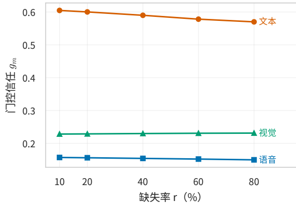
图 5.5 门控信任随缺失率的响应（验证集，三种子均值）
