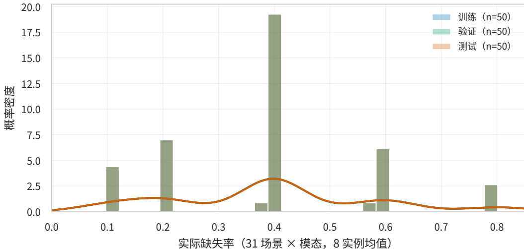
31 缺失场景实际缺失率分布 (train / valid / test)
