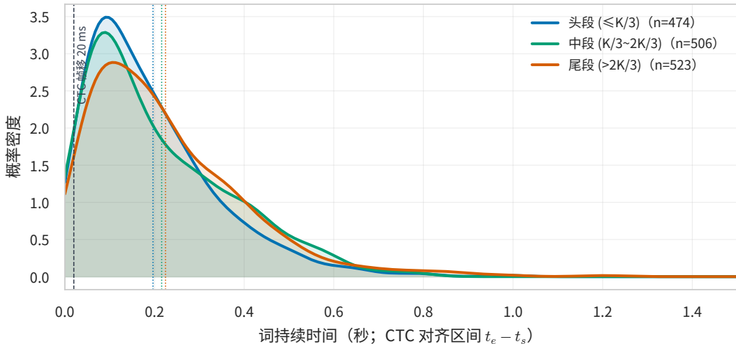
词持续时间按位置分位的核密度 (76 样本 \times 1503 词)
