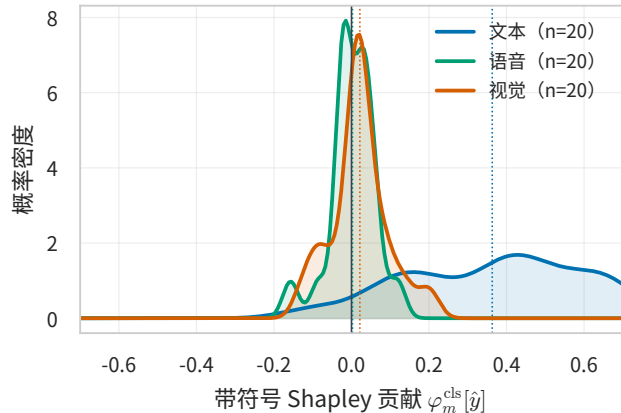
(a) 带符号贡献密度
