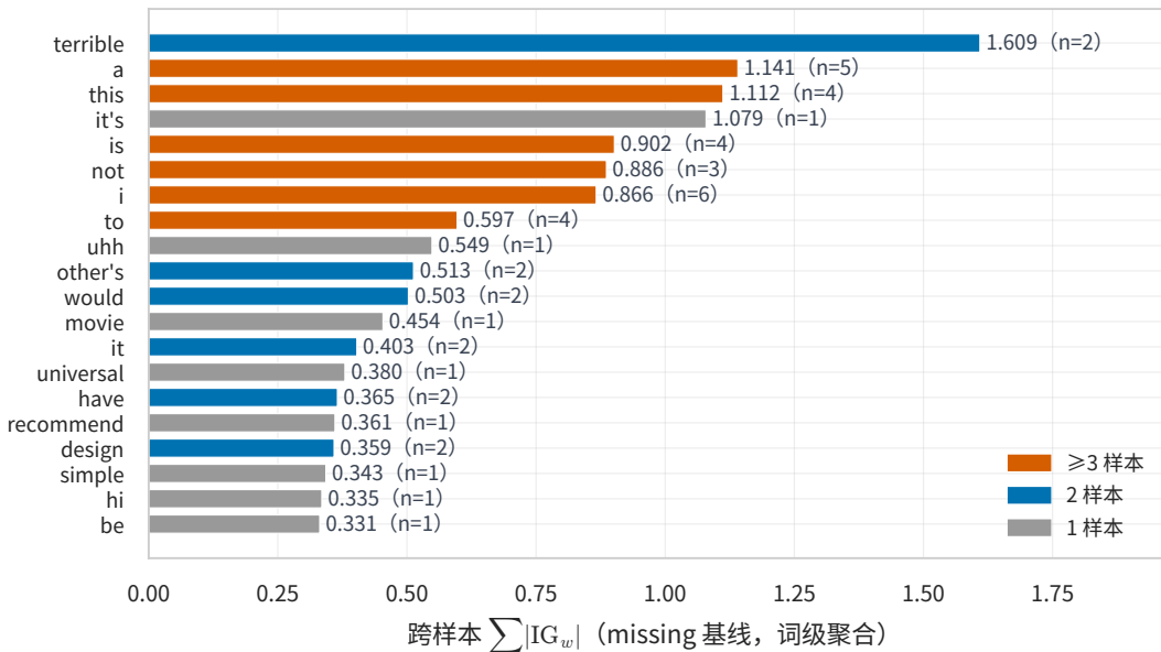
TOP-20 关键词 IG 贡献 (附件4, 20 样本词级聚合)
