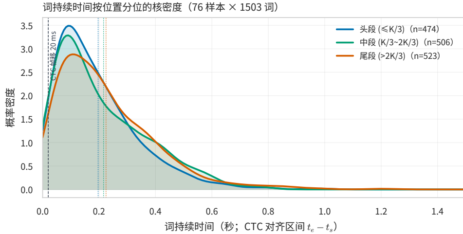
图 4.1 词持续时间按位置分位的核密度 (CTC 对齐区间)
