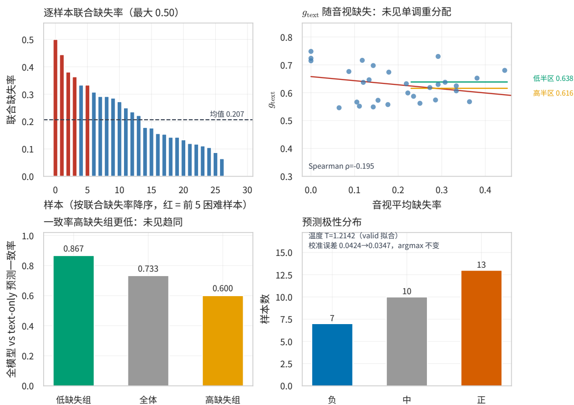
图 5.6 附件 3 行为分析（MRFN+ 集成，30 条，无标签）
