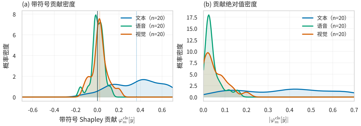
图 6.2 三模态 Shapley 贡献密度 (附件 4, n = 20 )
