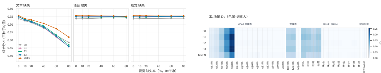
图 5.4 缺失场景实验：(a) 退化曲线 (b) 热力图
