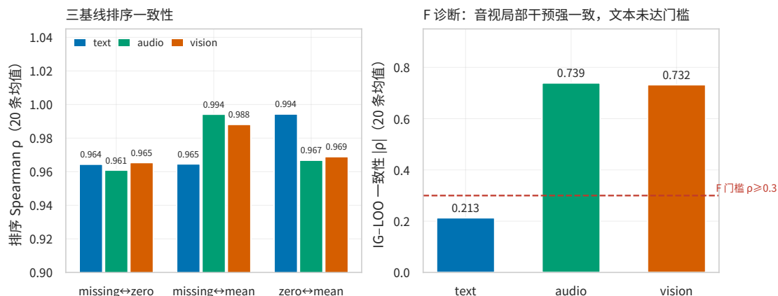
图 6.3 IG 验证与 F 项诊断 (三基线排序一致性)
