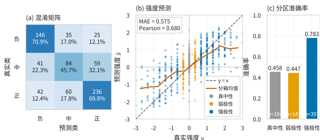
图 7.1 MRFN+ 双输出性能与误差结构
