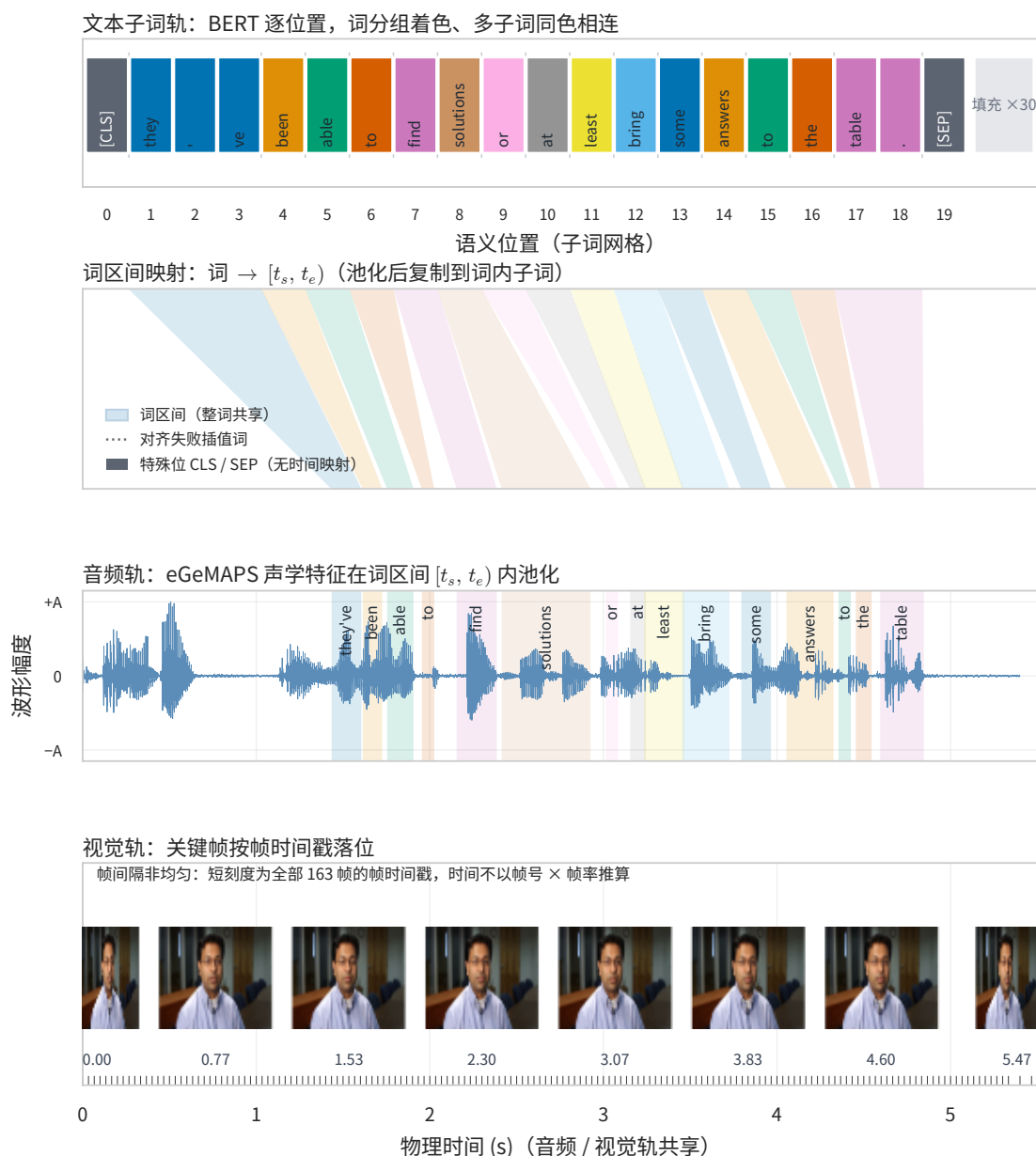
图 4.3 统一时序坐标图（文本位置域与物理时间域经词区间映射）
