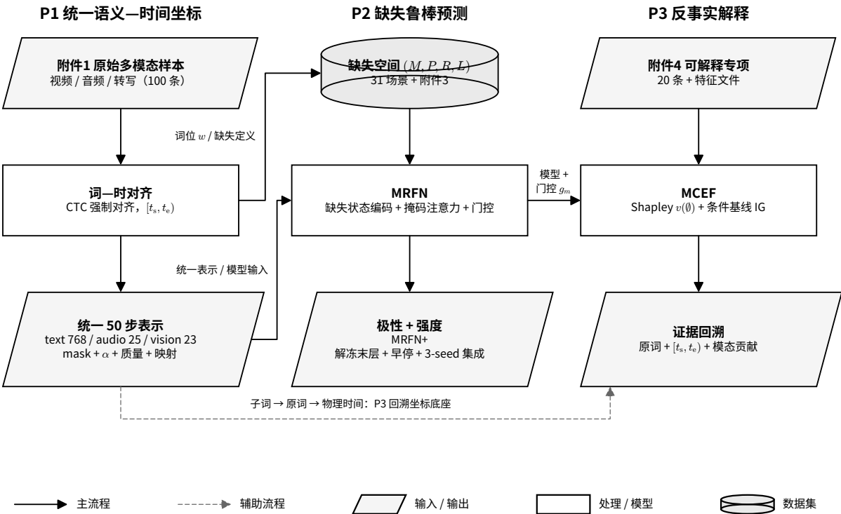
图 2.2 全文总体技术路线：统一坐标、鲁棒预测与反事实解释
