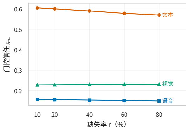
图 5.5 门控信任随缺失率的响应 (验证集, 三种子均值)
