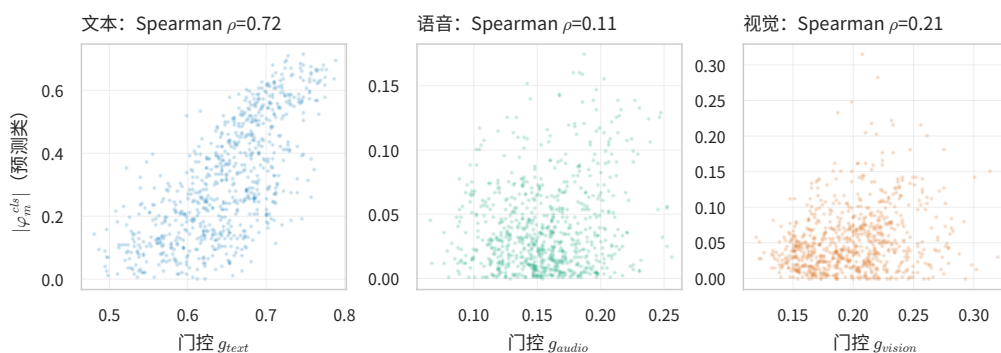
图 6.6 门控——贡献一致性散点（附件 2 验证集，728 条，分模态）
