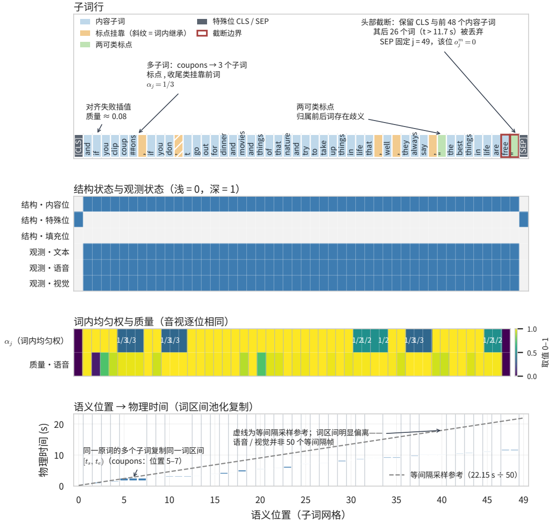
图 4.4 50 位语义网格与状态标注 (截断样本示例)
