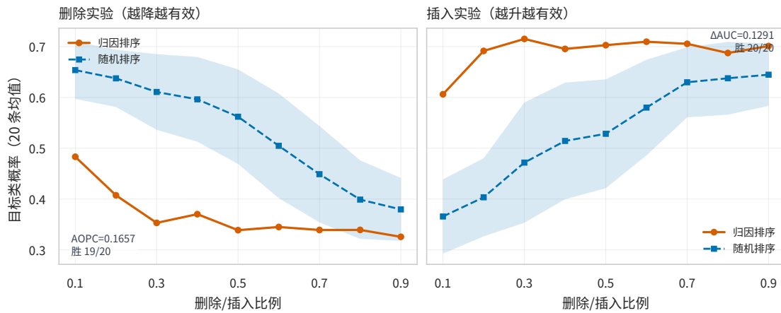
图 6.5 删除/插入保真度曲线（归因序与随机序对照）
