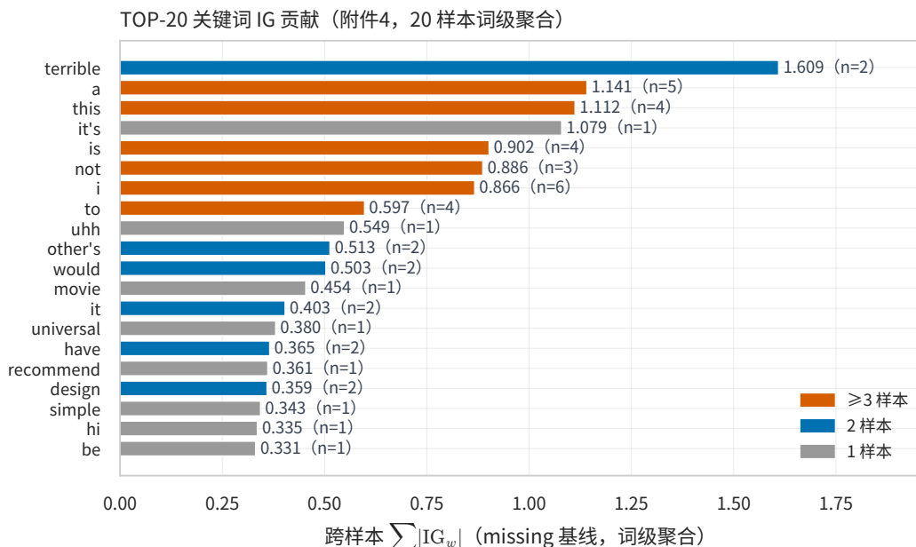
图 6.4 TOP-20 关键词 IG 贡献 (附件 4 词级聚合)
