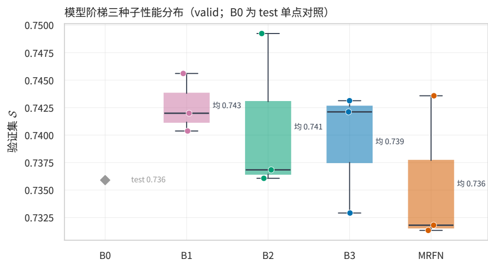
图 5.3 模型阶梯三种子重复性能分布（验证集，B0 为测试集对照）
