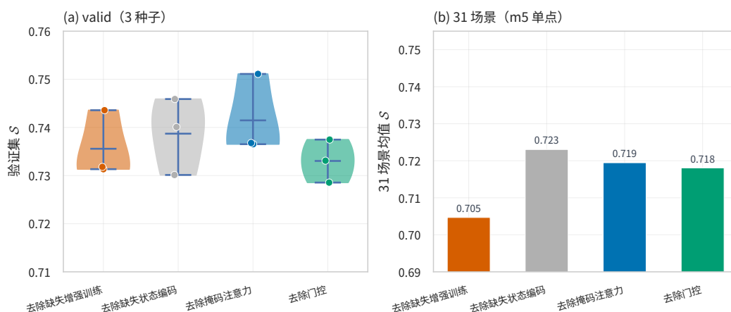
图 5.7 四项消融变体的性能分布
