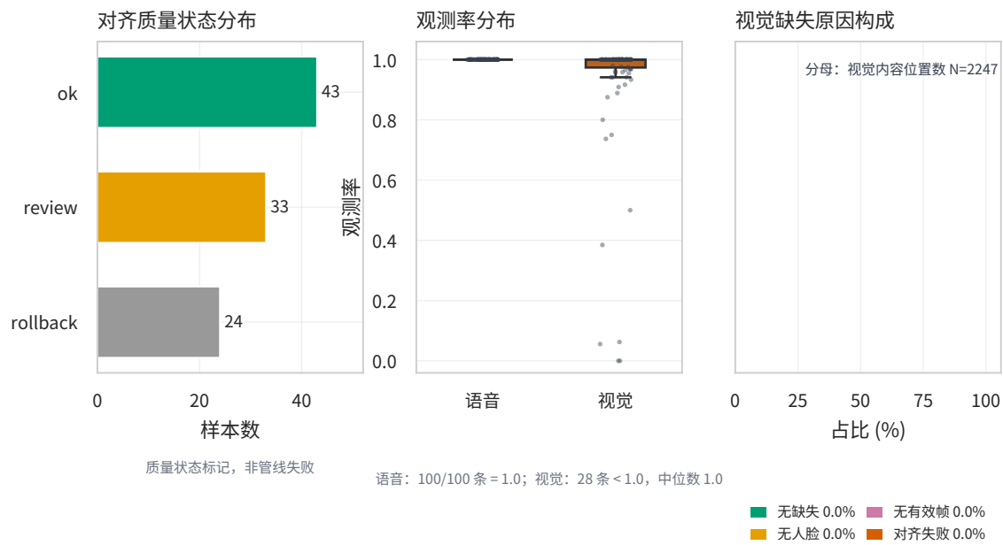
图 3.5 问题一验收三联图：对齐质量、观测率与缺失原因
