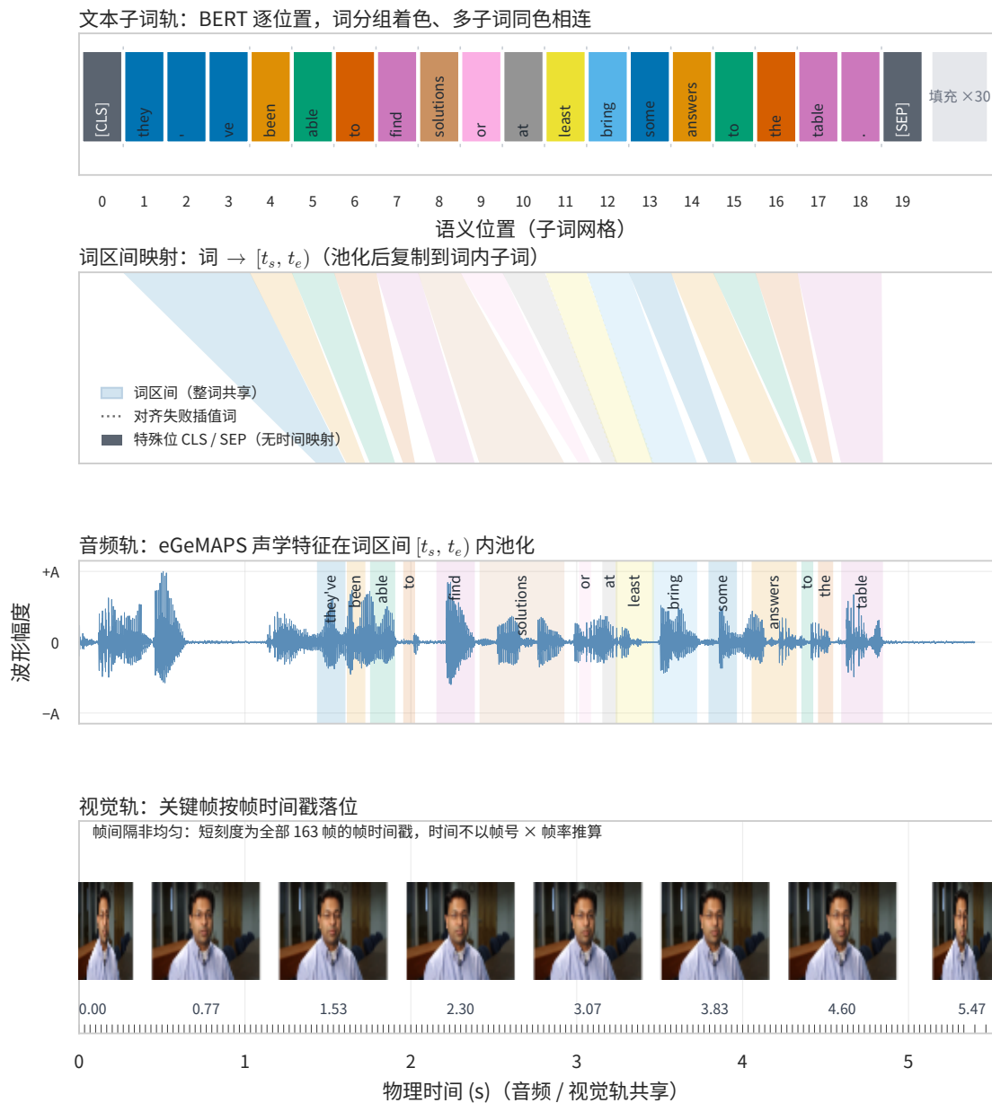
图 3.3 统一时序坐标图（文本位置域与物理时间域经词区间映射）
