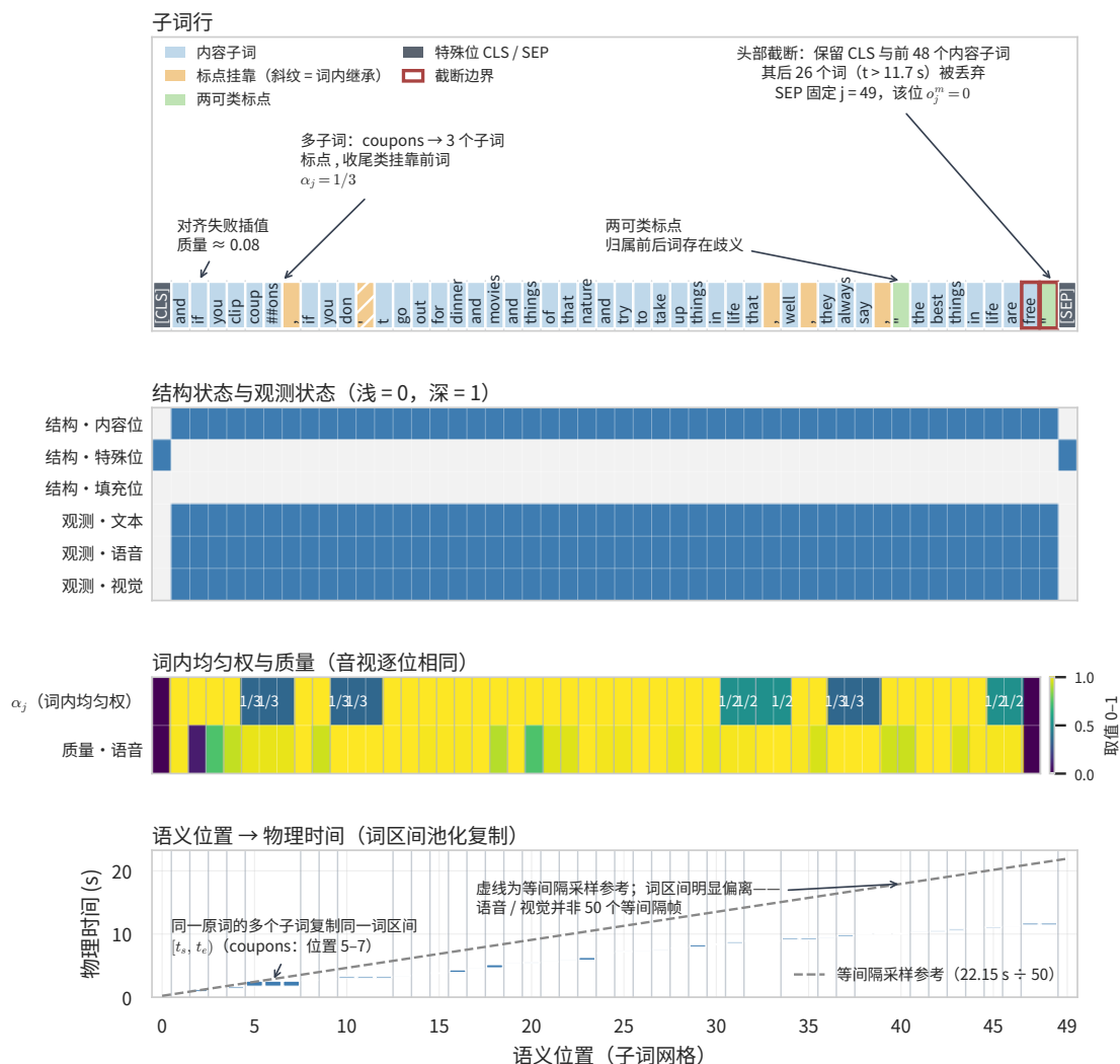
图 3.4 50 位语义网格与状态标注（截断样本示例）
