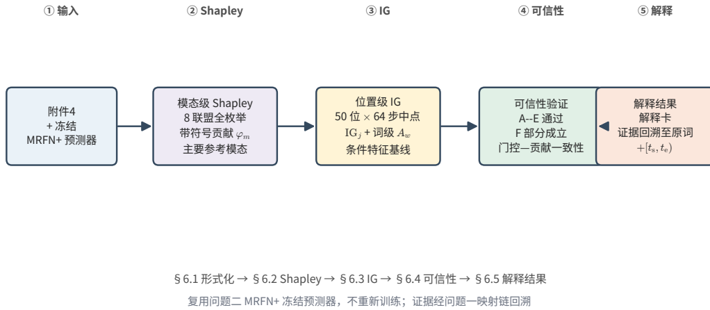
图 6.11 问题三求解流程：解释任务形式化 → 模态级 Shapley → 位置级 IG → 六项保真度检验 → 附件 4 证据回溯
