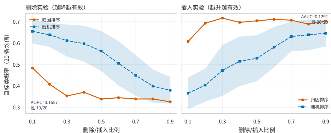
图 6.14 删除/插入保真度曲线（归因序与随机序对照）
