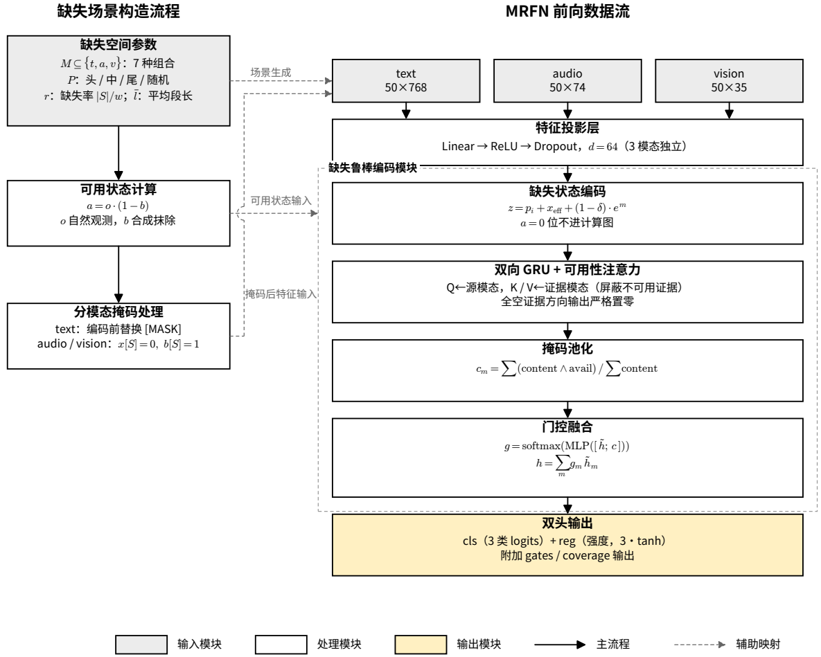
图 4.7 MRFN 缺失场景构造与数据流（左：三级构造；右：四阶段）
