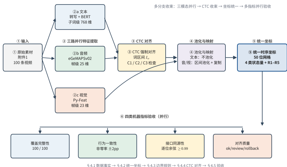
图 3.2 问题一求解流程：原始素材 → 子词化与特征提取 → CTC 强制对齐 → 统一时序坐标 → 四类机器指标验收
