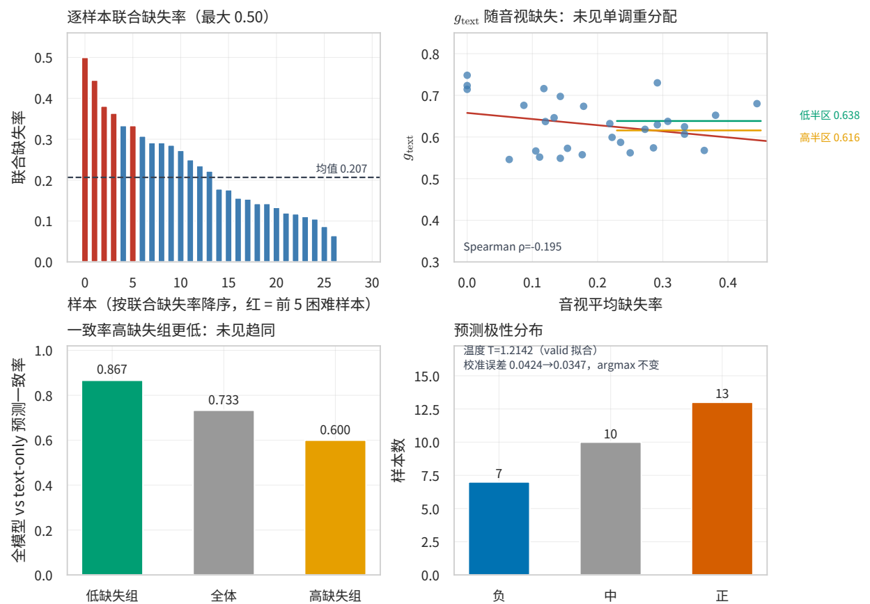
图 4.10 附件 3 行为分析（MRFN+ 集成，30 条，无标签）
