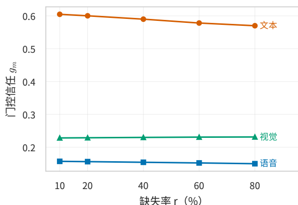
图 4.9 门控信任随缺失率的响应 (验证集, 三种子均值)
