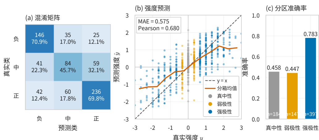
图 6.17 MRFN+ 双输出性能与误差结构（附件 2 验证集，728 条）
