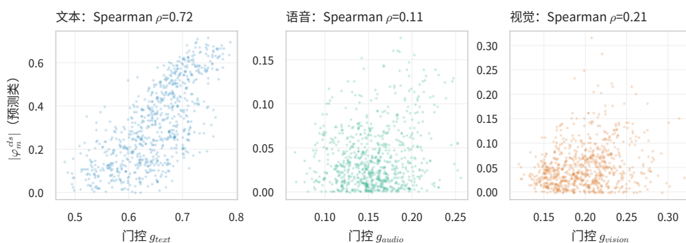
图 6.15 门控——贡献一致性散点（附件 2 验证集，728 条，分模态）
