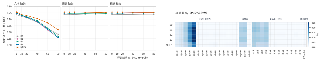
图 4.8 缺失场景实验结果: (a) 退化曲线; (b) D_S 热力图
