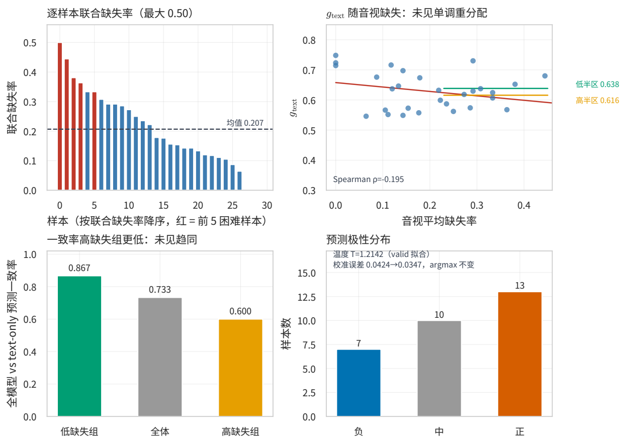
图 5.8 附件 3 行为分析（MRFN+ 集成，30 条，无标签）
