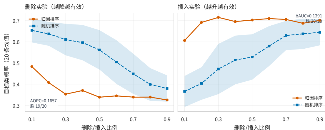
图 6.11 删除/插入保真度曲线（归因序与随机序对照）
