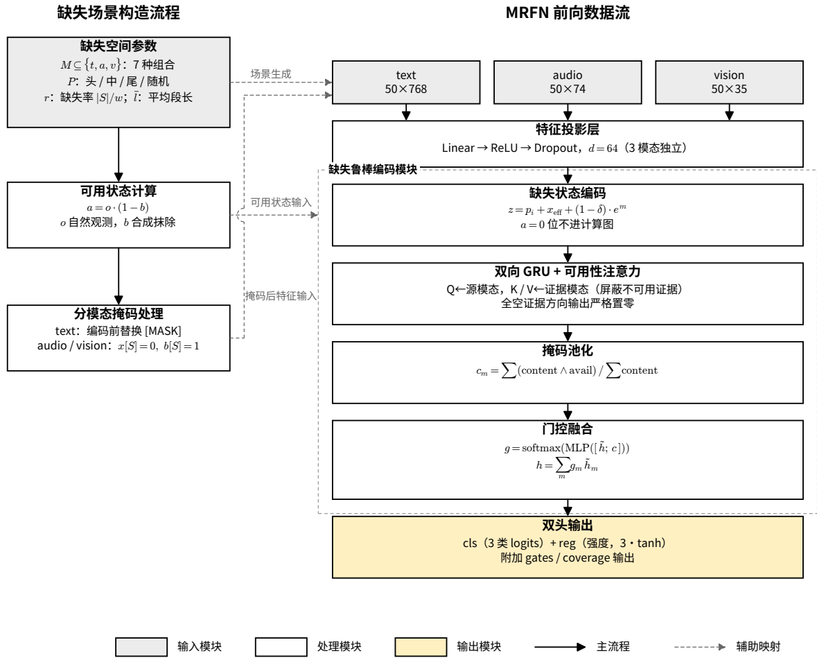
图 5.5 MRFN 缺失场景构造与数据流（左：三级构造；右：四阶段）
