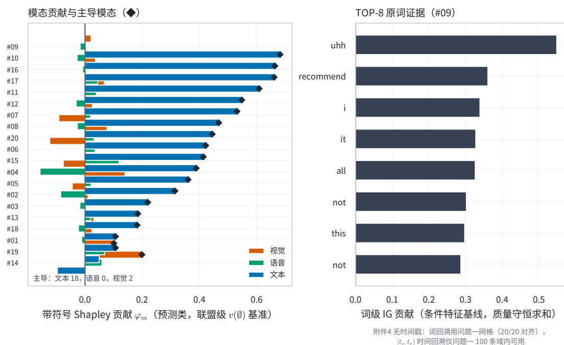
图 6.9 模态贡献与词级证据回溯 (附件 4, 20 条)
