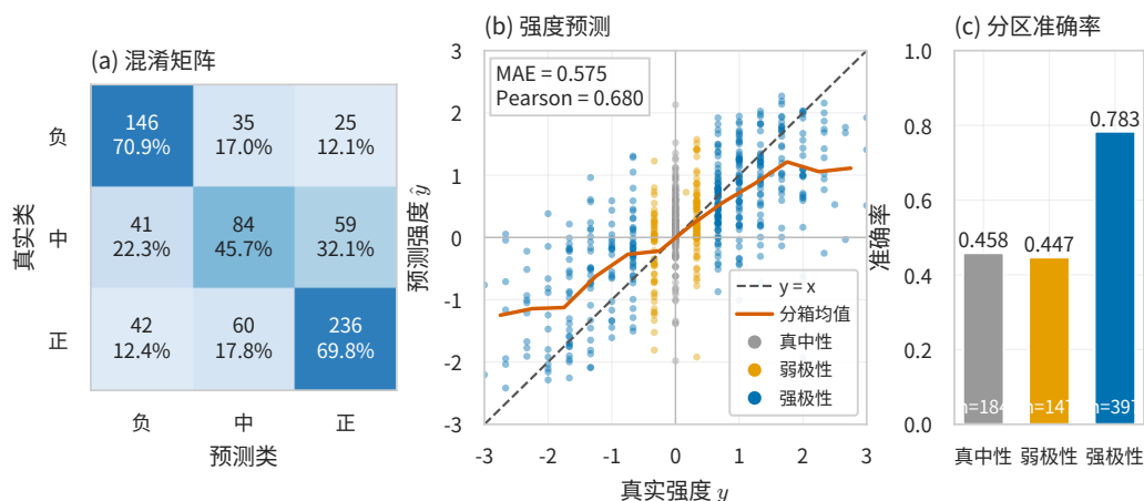
图 7.14 MRFN+ 双输出性能与误差结构（附件 2 valid，728 条）
