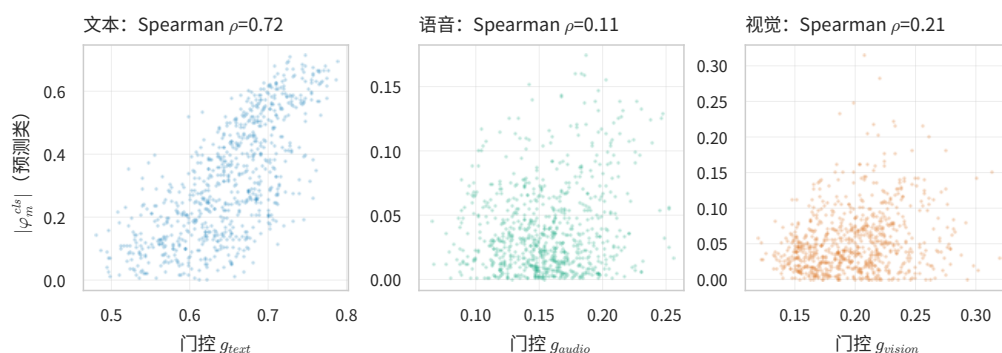
图 6.12 门控——贡献一致性散点（附件 2 valid，728 条，分模态）
