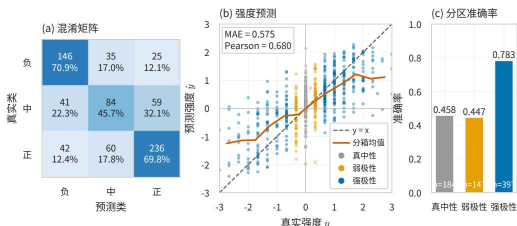
图 6.16 MRFN+ 双输出性能与误差结构（附件 2 验证集，728 条）
