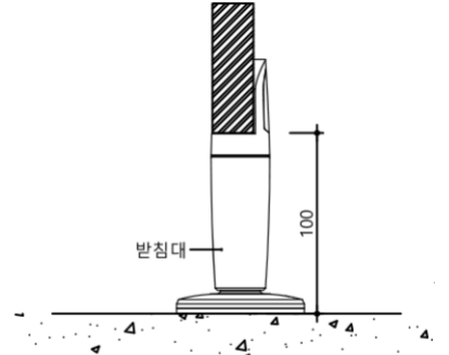
받침대 (측면부)
