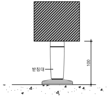
받침대 (전면부)
