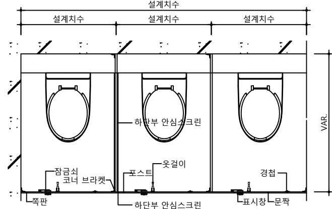
평면도
