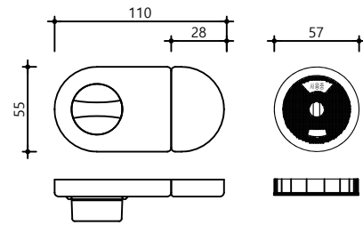
하드웨어 - 잠금쇠
