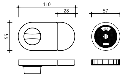
하드웨어 - 잠금쇠
