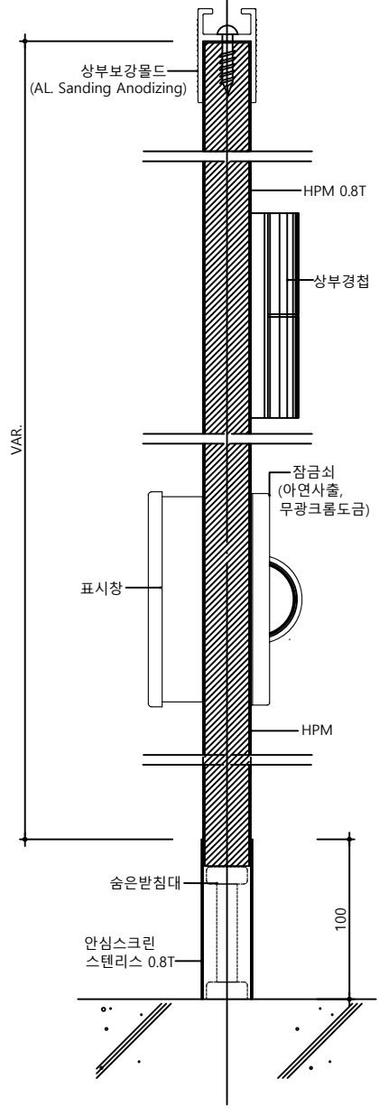
단면도 축척 : NONE
