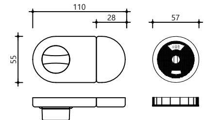
하드웨어 - 잠금쇠
