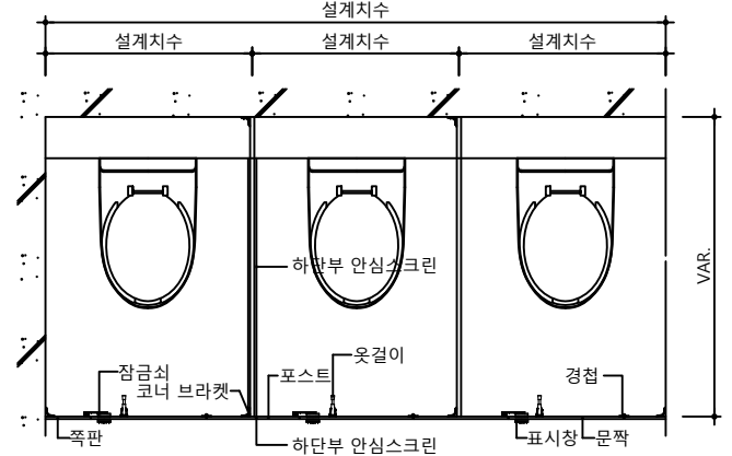
평면도
