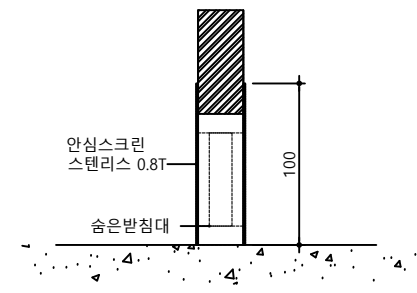
안심스크린(측면부)
