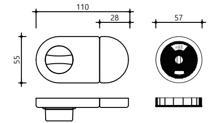
하드웨어 - 잠금쇠
