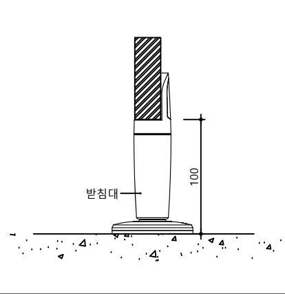
받침대 (측면부)
