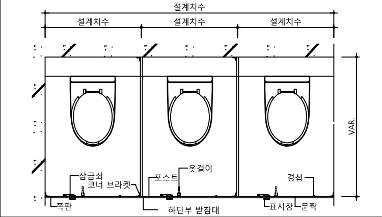
평면도
