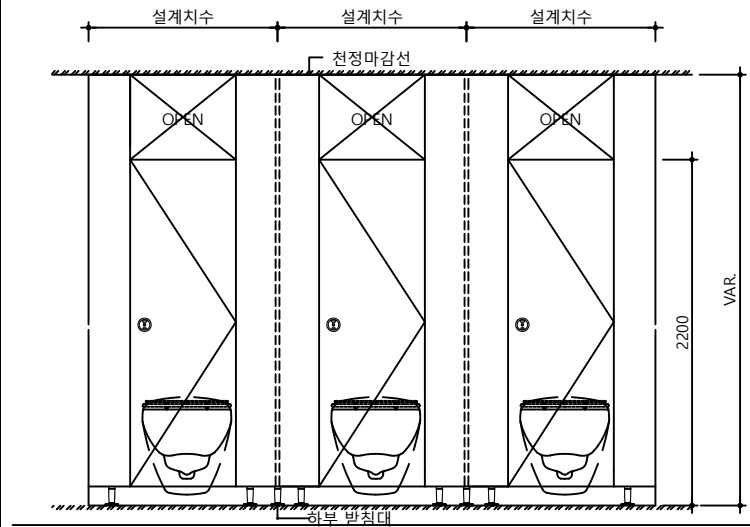
입면도 TYPE A
