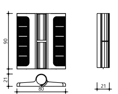
하드웨어 - 경첩
