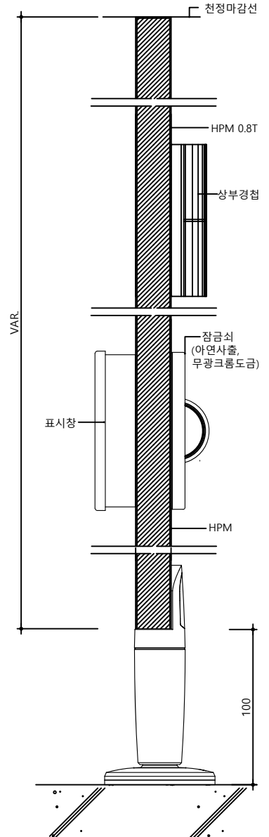
단면도 축척 : NONE
