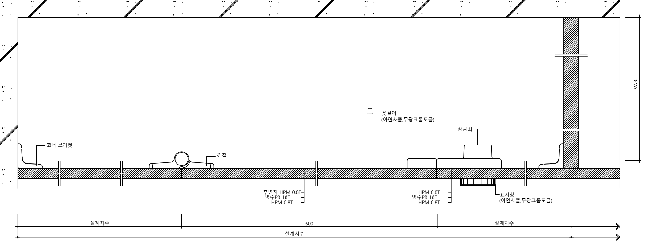
판넬 상세도 축척 : NONE
