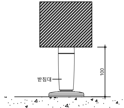
받침대 (전면부)
