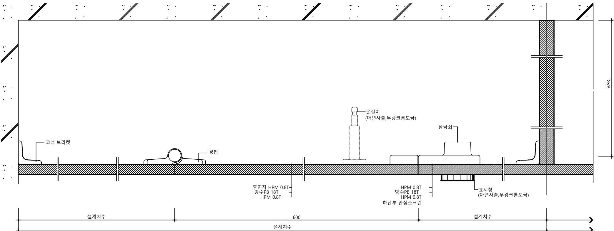
판넬 상세도 축척 : NONE
