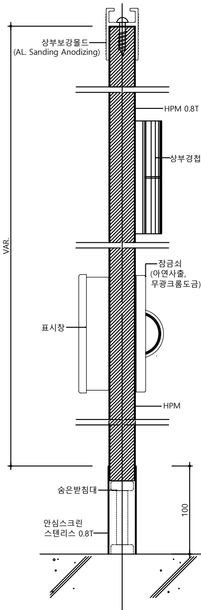
단면도 축척 : NONE
