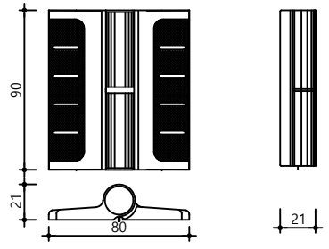
하드웨어 - 경첩
