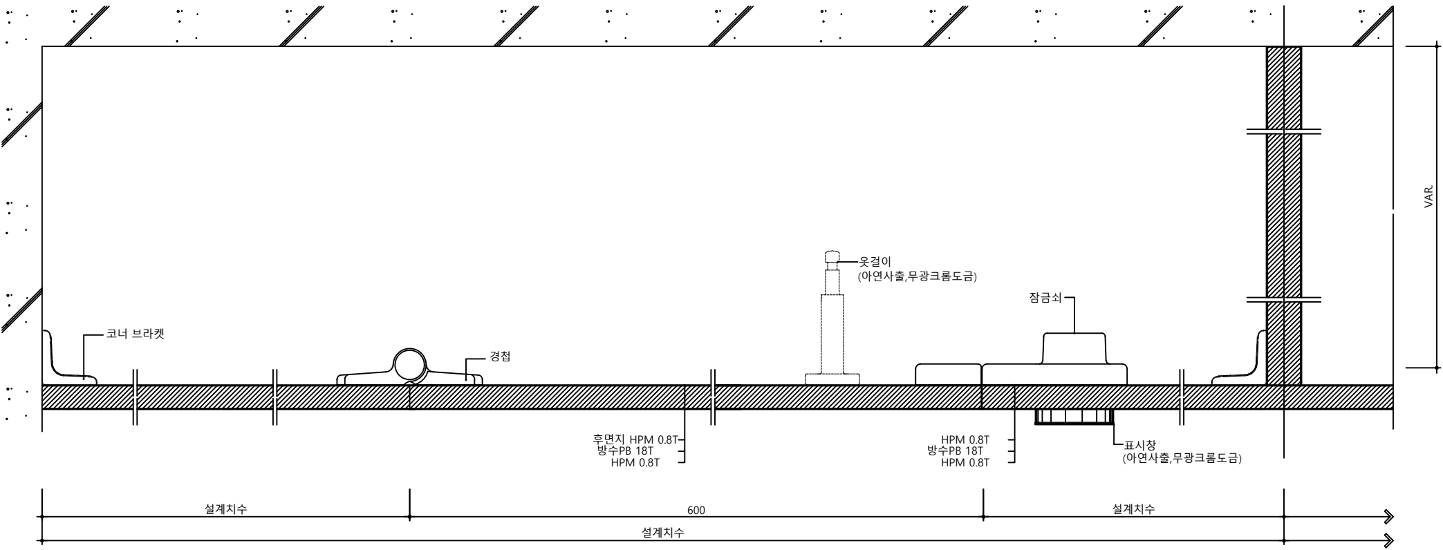
판넬 상세도
