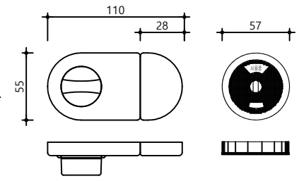
하드웨어 - 잠금쇠
