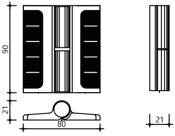
하드웨어 - 경첩
