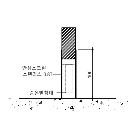
안심스크린 상세(전면부)
