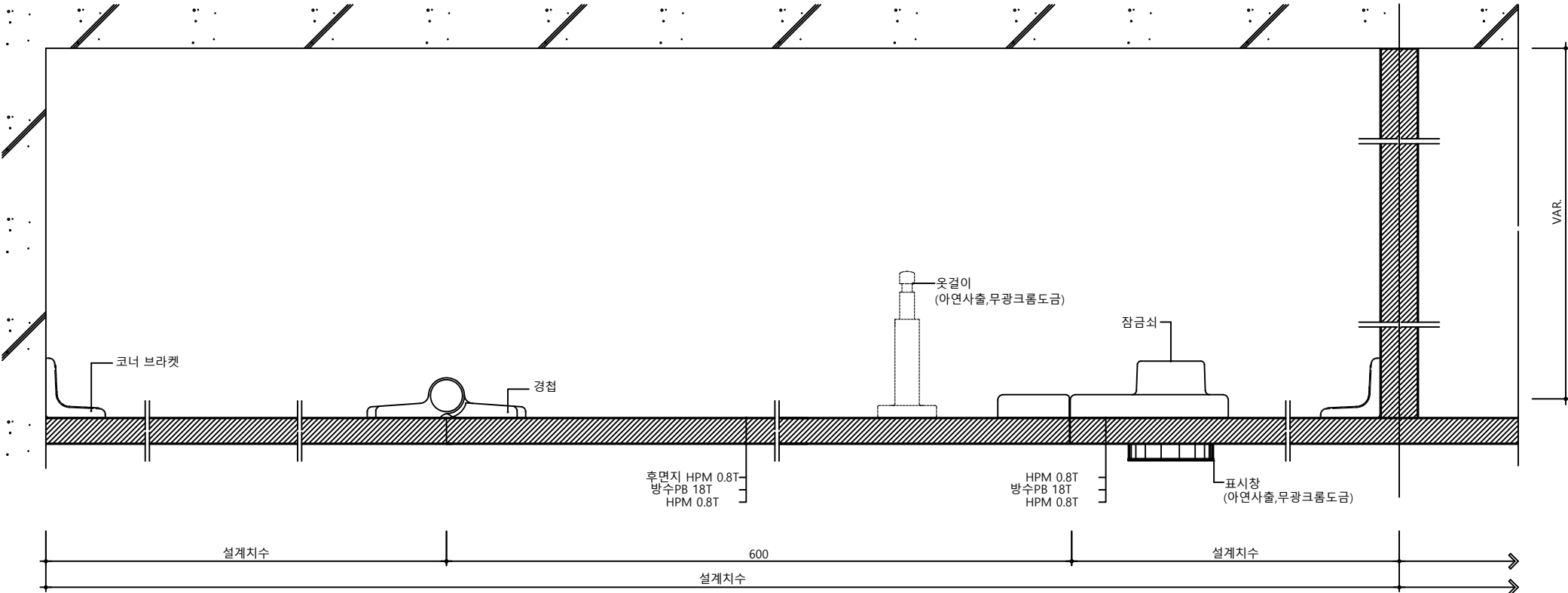
판넬 상세도
