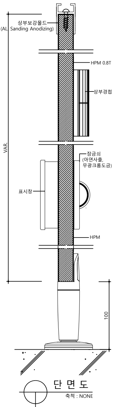
하드웨어 - 잠금쇠
