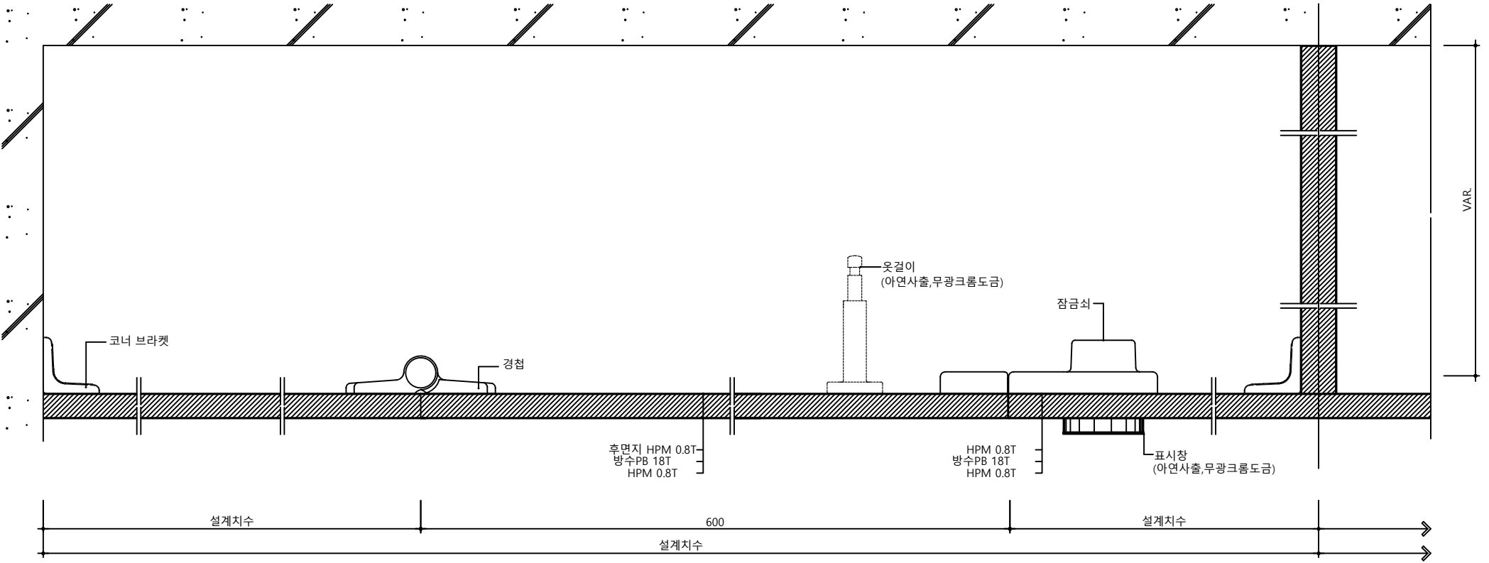
판넬 상세도
