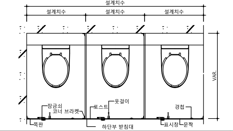
평면도
