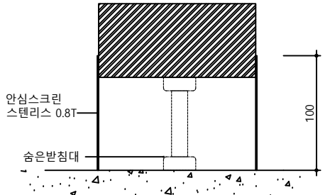
안심스크린 상세(전면부)
