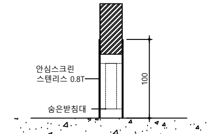
안심스크린(측면부)
