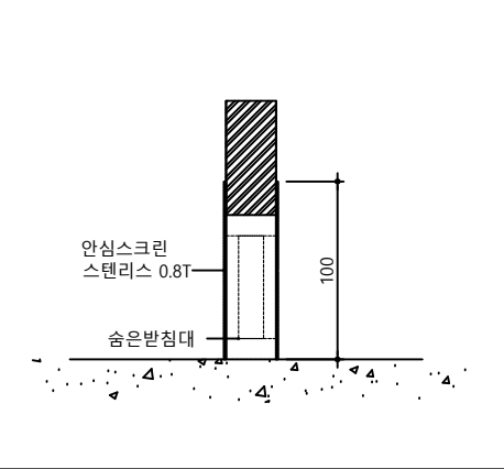
안심스크린(측면부)
