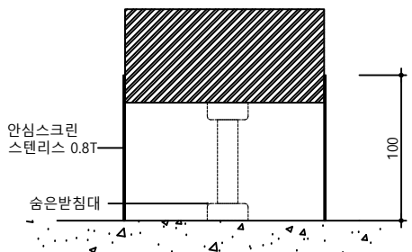
안심스크린 상세(전면부)
