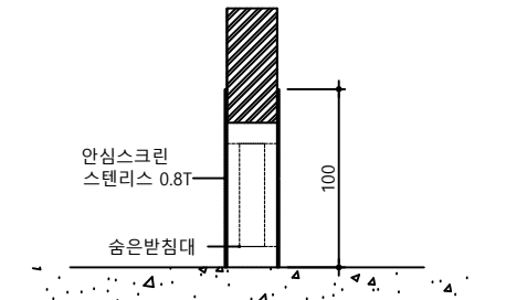
안심스크린(측면부)
