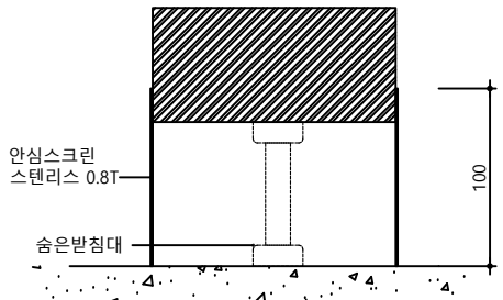
안심스크린 상세(전면부)
