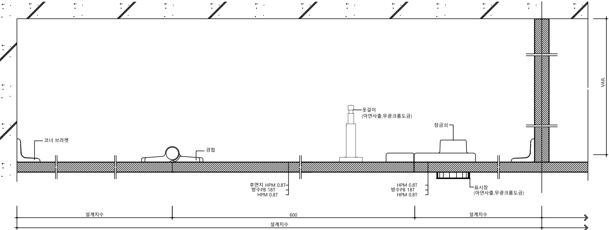
판넬 상세도
