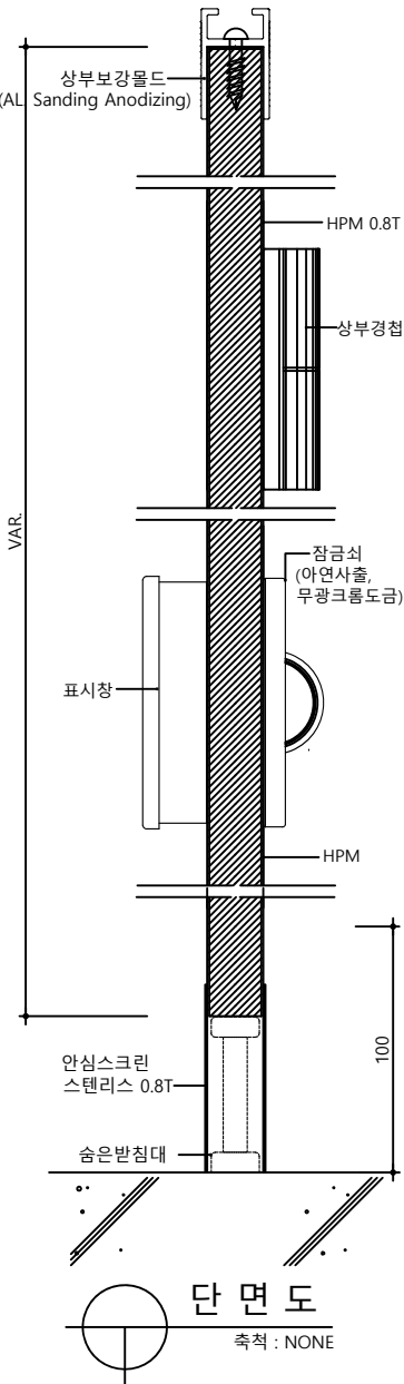
하드웨어 - 잠금쇠
