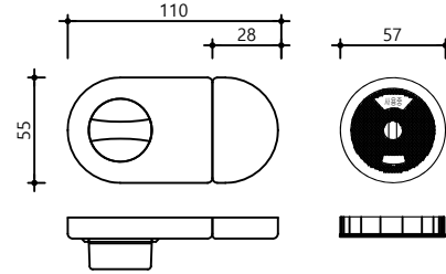
하드웨어 - 잠금쇠
