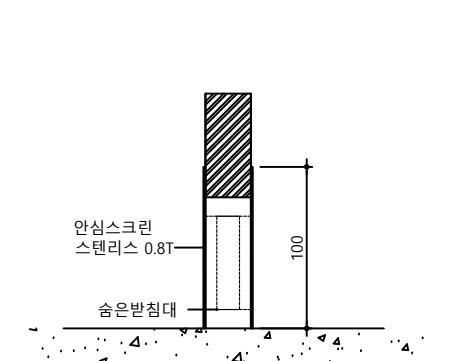
안심스크린 상세(전면부)
