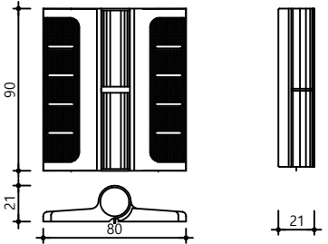
하드웨어 - 경첩
