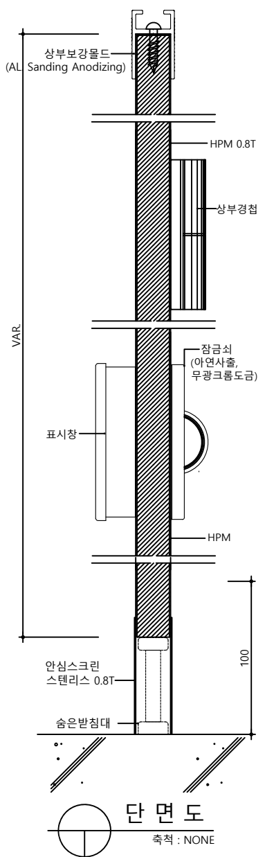
하드웨어 - 잠금쇠
