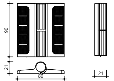
하드웨어 - 경첩
