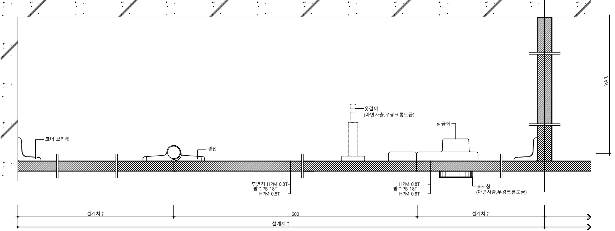
판넬 상세도
