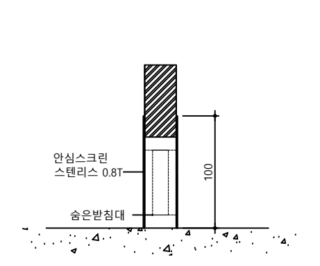
안심스크린 상세(전면부)
