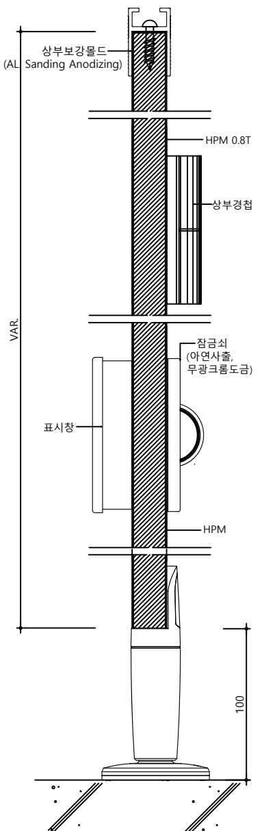
단면도
