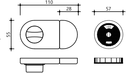
하드웨어 - 잠금쇠
