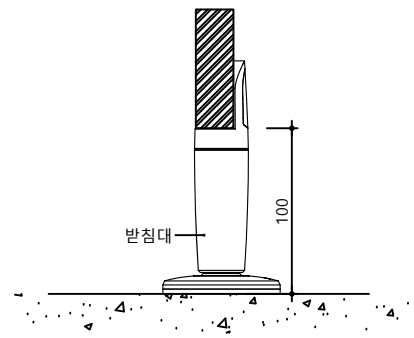
받침대 (측면부)
